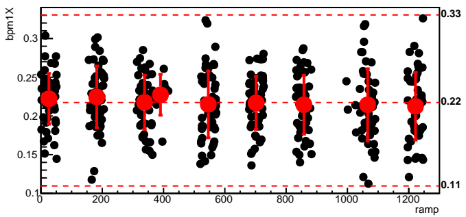
bmod_trim2,cyc=7495
