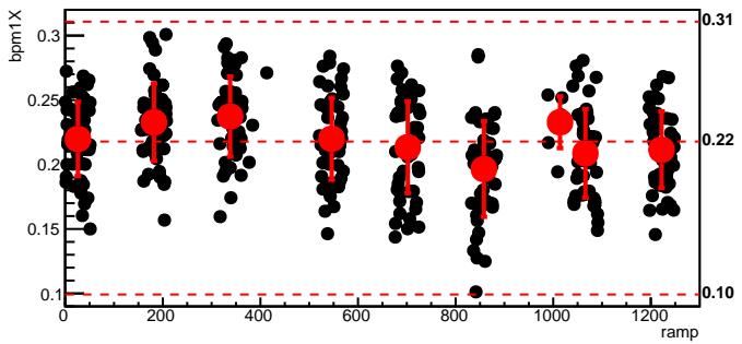
bmod_trim7,cyc=7495
