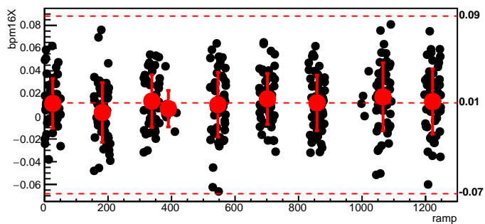
bmod_trim2,cyc=7495
