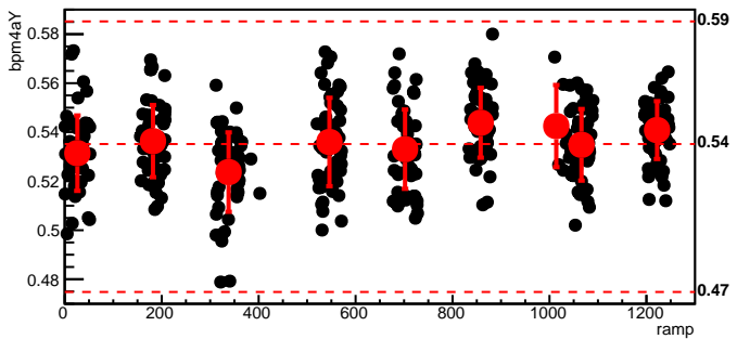
bmod_trim7,cyc=7495
