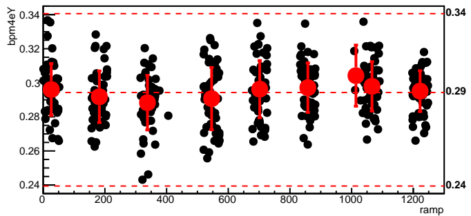
bmod_trim7,cyc=7495
