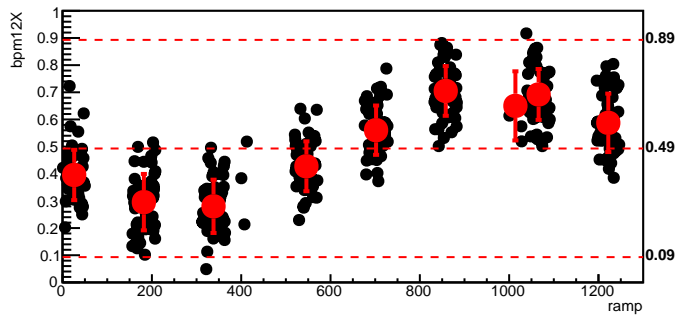
bmod_trim7,cyc=7495
