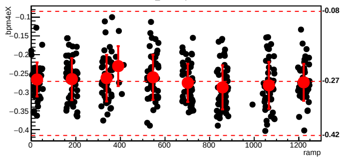
bmod_trim7,cyc=7587
