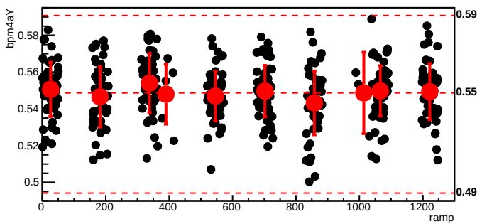
bmod_trim1,cyc=7587
