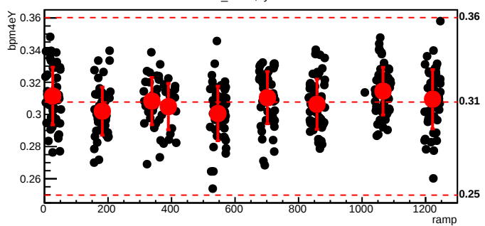
bmod_trim5,cyc=7587
