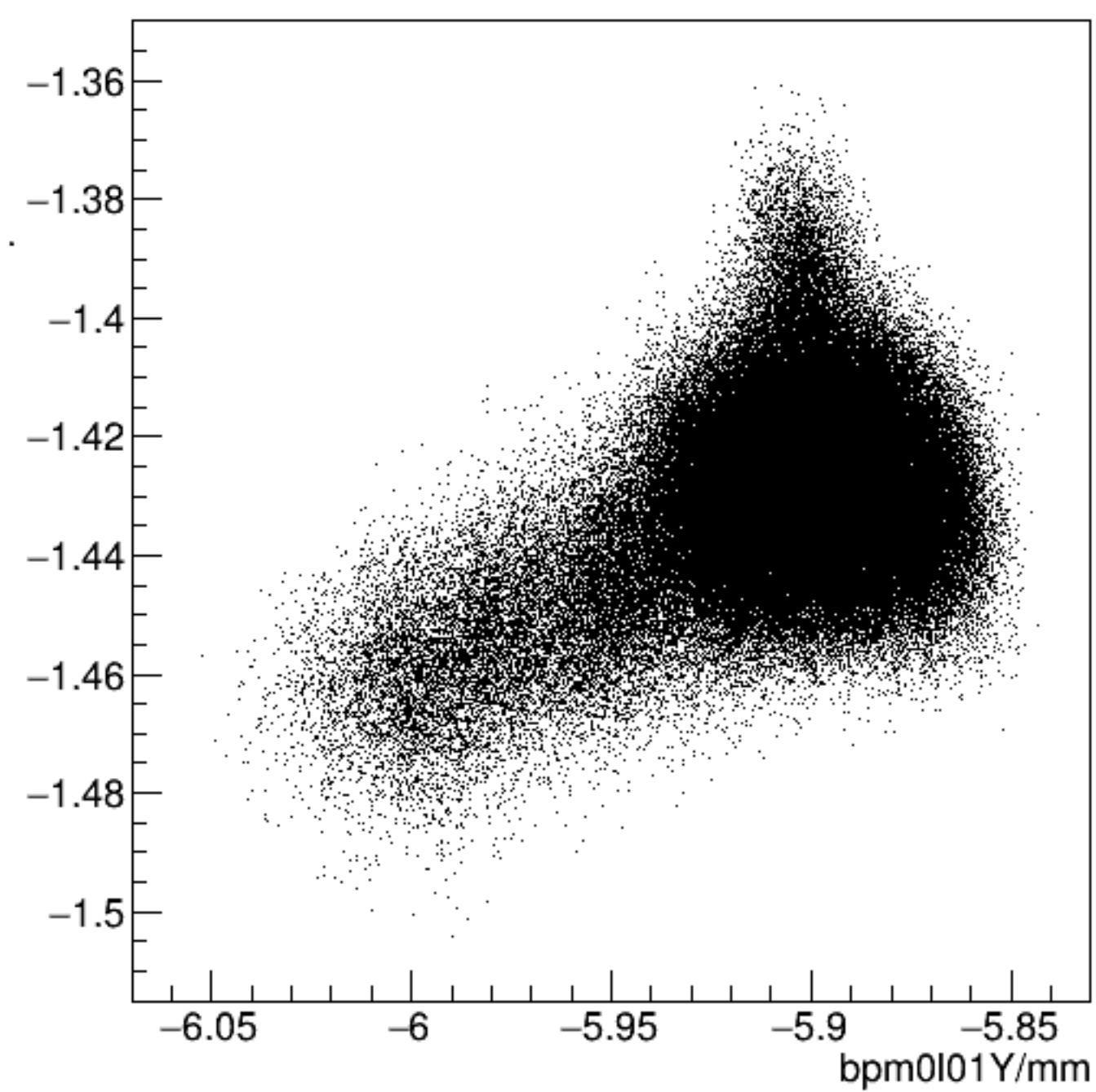
bpm0l01X/mm:bpm0l01Y/mm {ErrorFlag==0}
