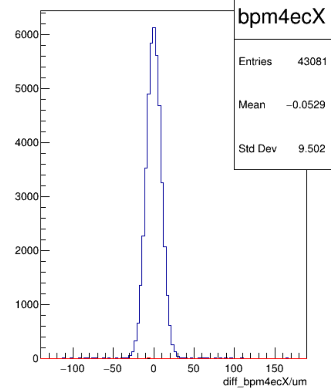
diff_bpm4ecX/um (ErrorFlag==0)
