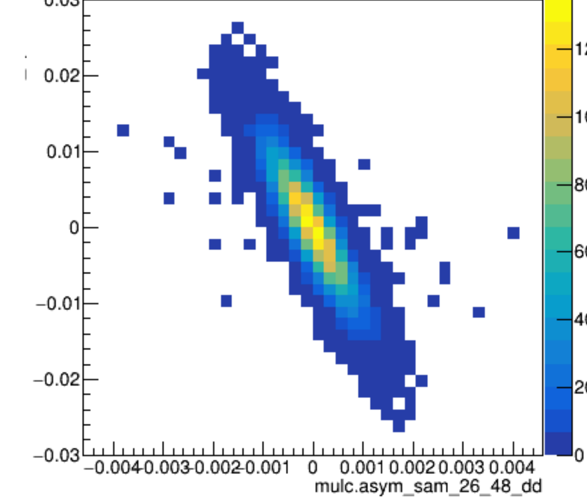
asym_sam_26_48_dd
