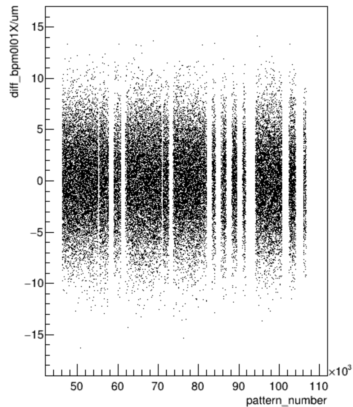
diff_bpm0l01X/um:pattern_number (ErrorFlag==0)
