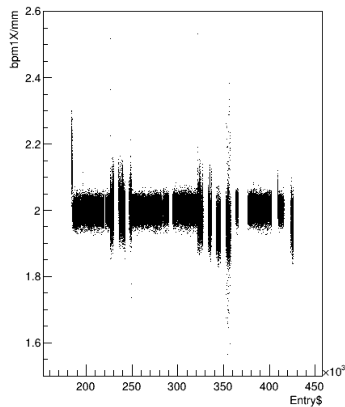
bpm1X/mm:Entry$ {ErrorFlag==0}
