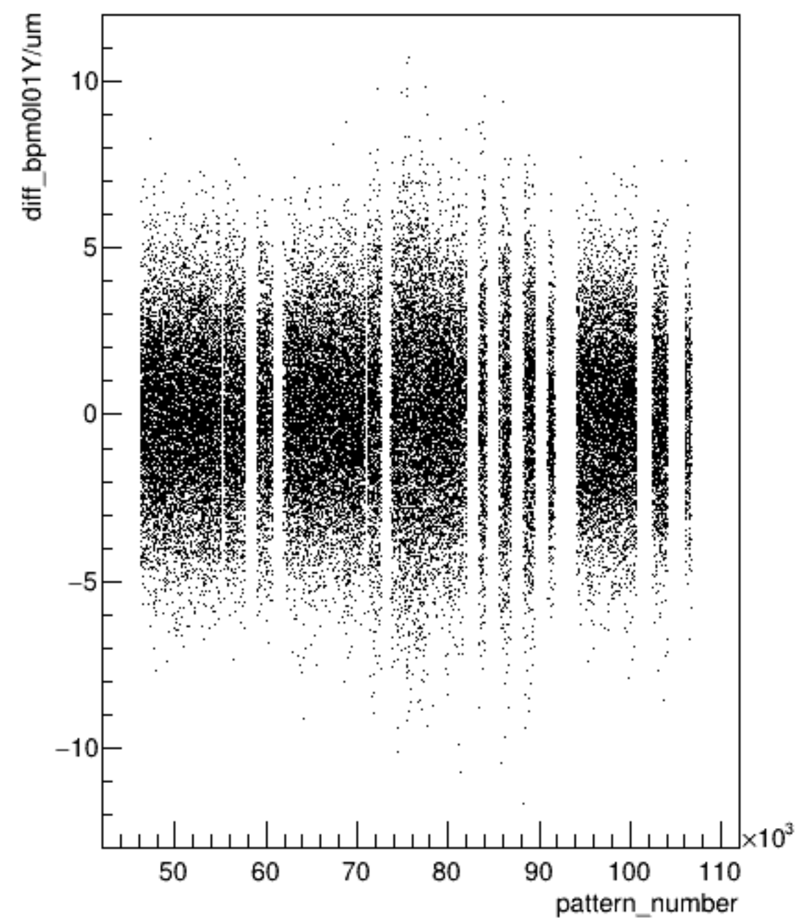
diff_bpm0l01Y/um:pattern_number (ErrorFlag==0)
