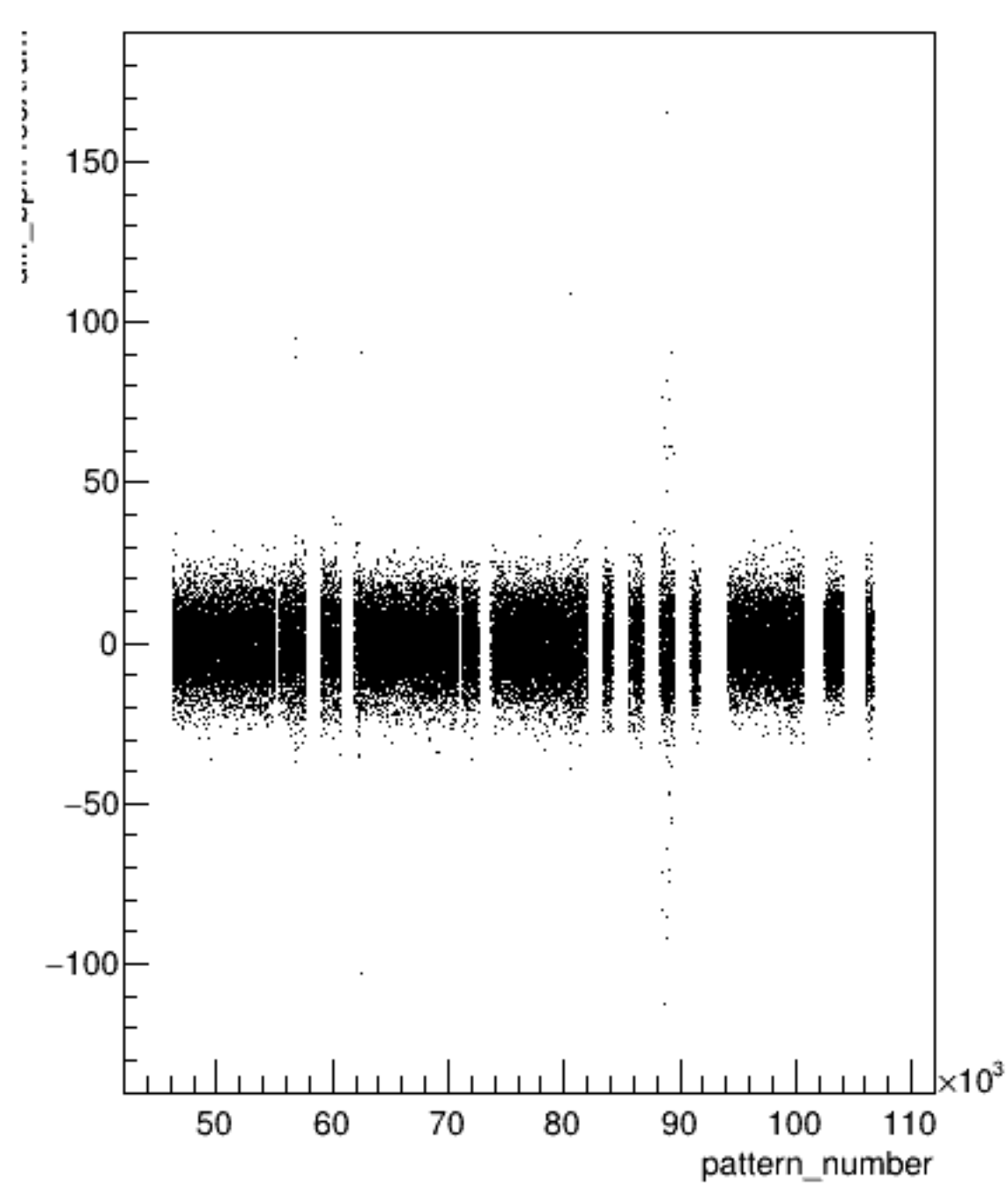
diff_bpm4ecX/um:pattern_number (ErrorFlag==0)
