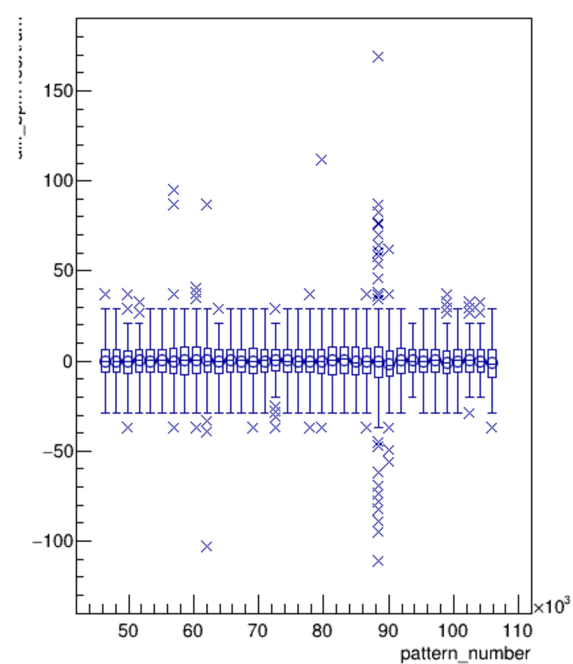
diff_bpm4ecX/um:pattern_number (ErrorFlag==0)
