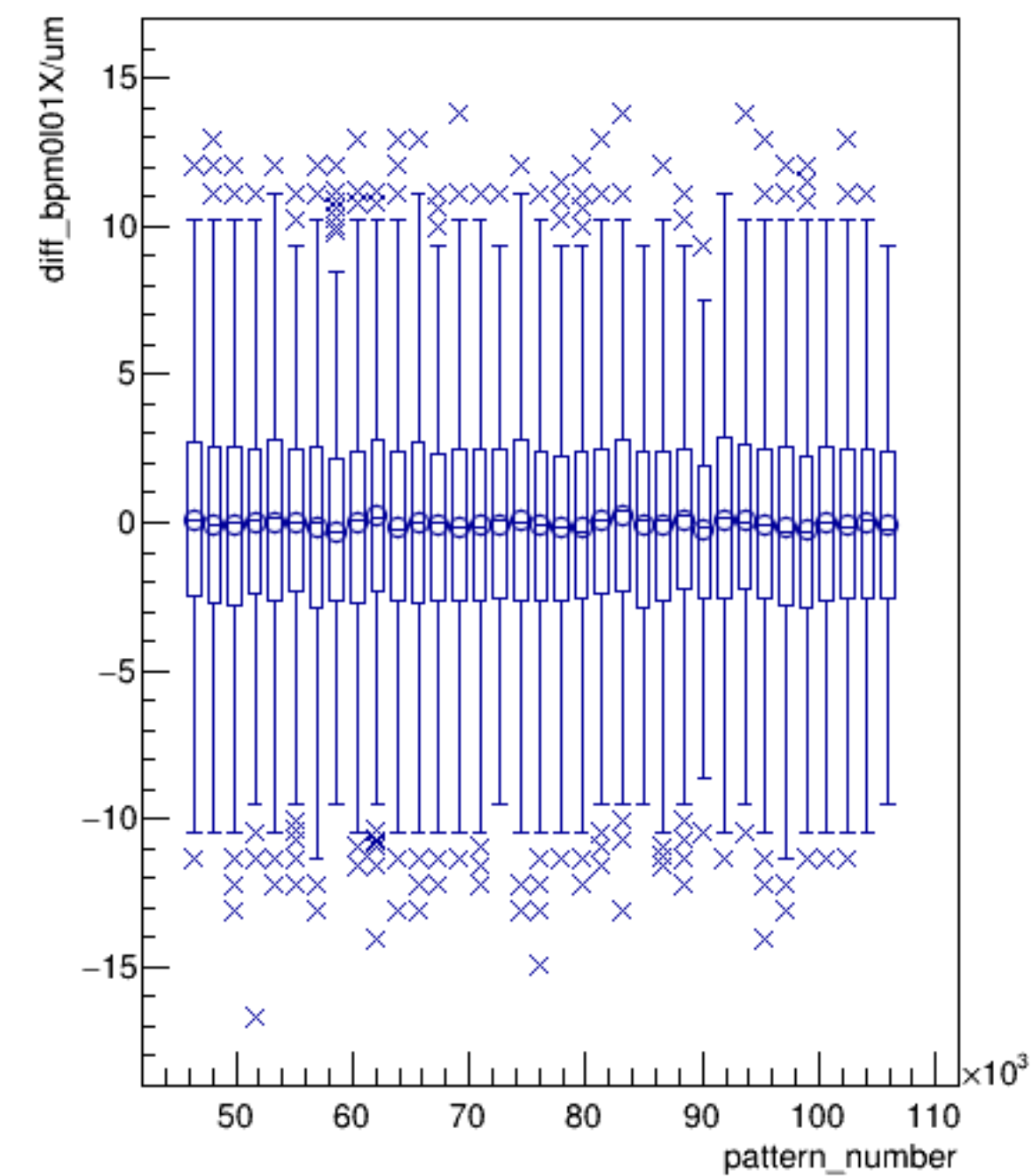
diff_bpm0l01X/um:pattern_number (ErrorFlag==0)
