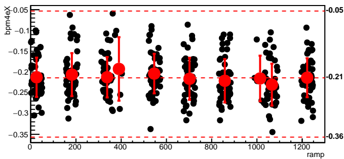
bmod_trim2,cyc=7628
