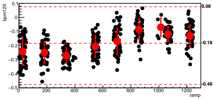
bmod_trim1,cyc=7628
