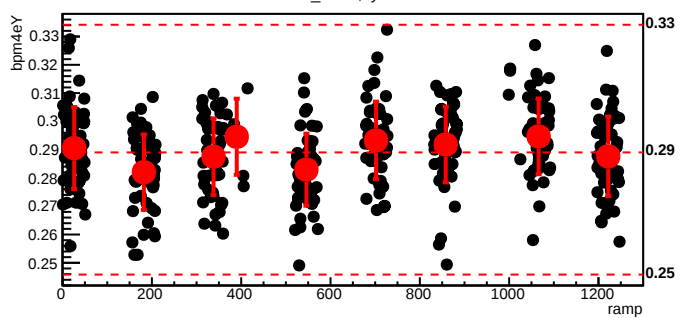
bmod_trim7,cyc=7662
