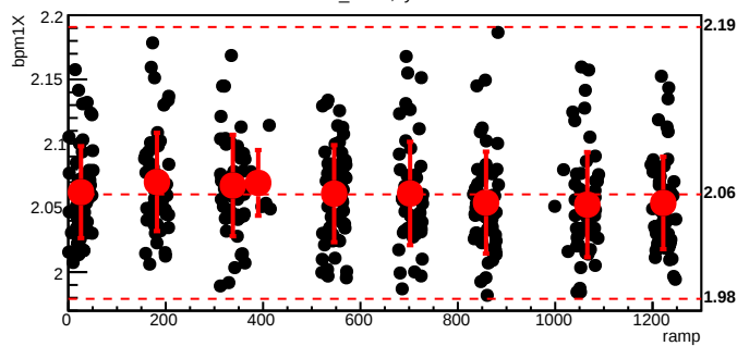
bmod_trim7,cyc=7662
