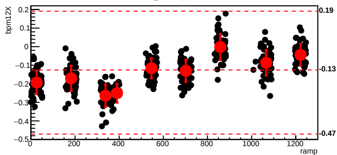
bmod_trim1,cyc=7675
