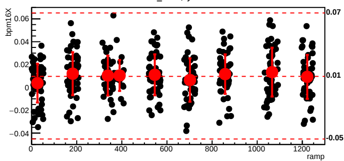
bmod_trim6,cyc=7675
