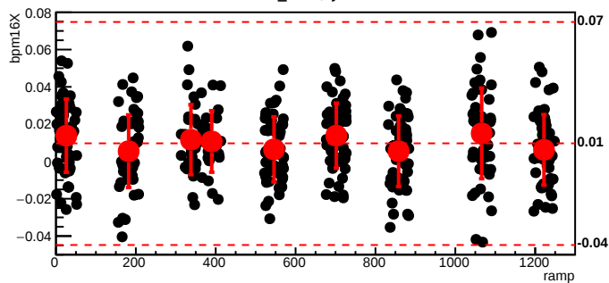
bmod_trim4,cyc=7675
