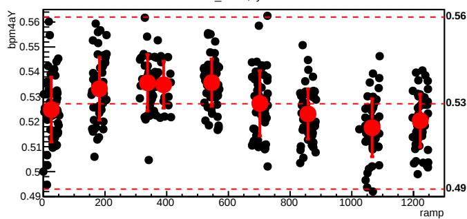
bmod_trim3,cyc=7675
