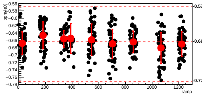
bmod_trim7,cyc=7675
