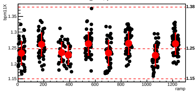
bmod_trim4,cyc=7675
