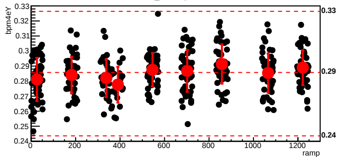
bmod_trim7,cyc=7675
