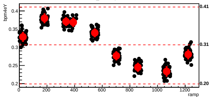
bmod_trim2,cyc=7675
