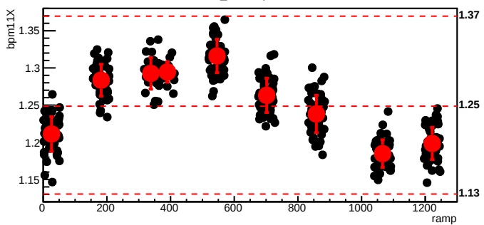
bmod_trim5,cyc=7675
