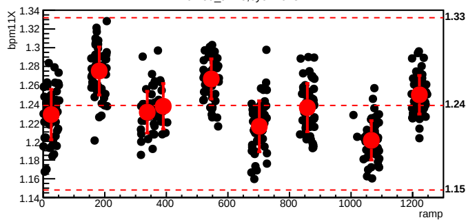
bmod_trim6,cyc=7675
