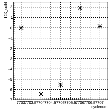
run:cyclenum {run == 7015}
