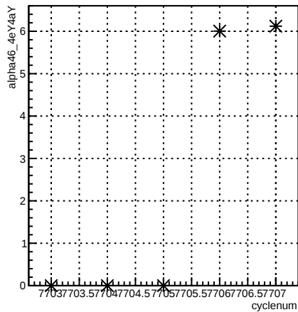
run:cyclenum {run == 7015}
