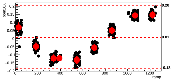
bmod_trim5,cyc=7703
