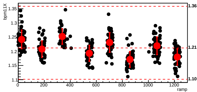
bmod_trim6,cyc=7703
