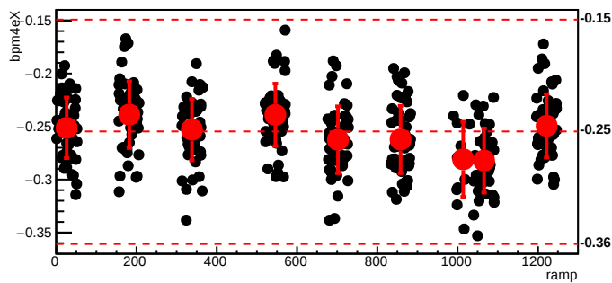
bmod_trim7,cyc=7703
