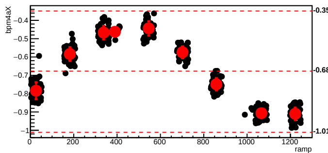
bmod_trim5,cyc=7703
