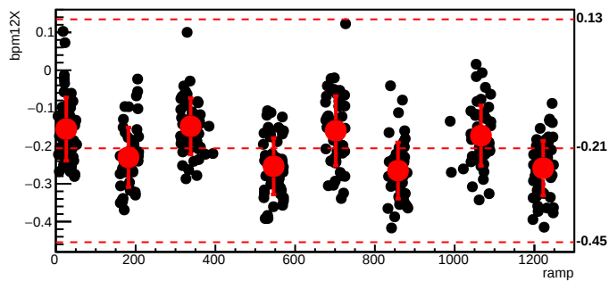
bmod_trim6,cyc=7703
