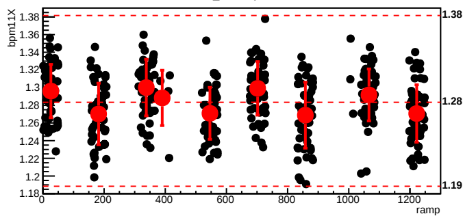
bmod_trim4,cyc=7804
