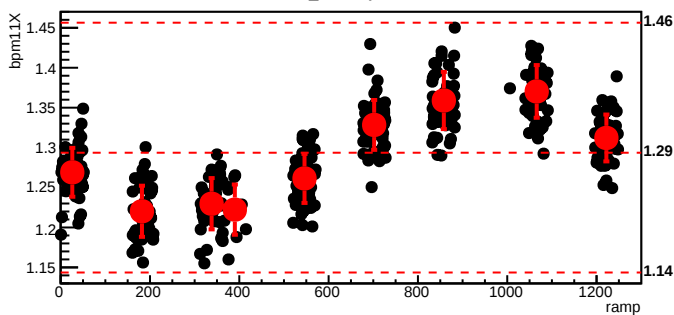
bmod_trim7,cyc=7804
