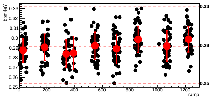
bmod_trim7,cyc=7804
