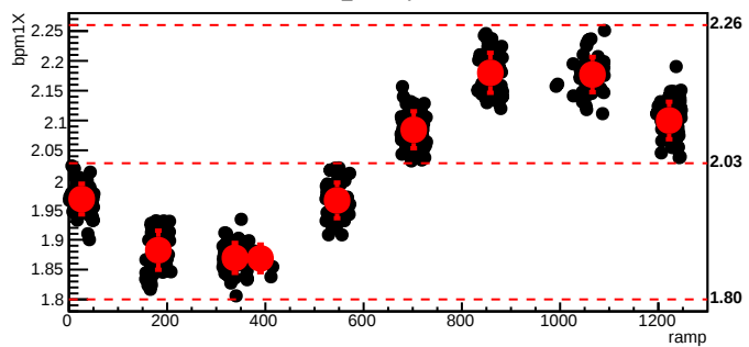
bmod_trim1,cyc=7804
