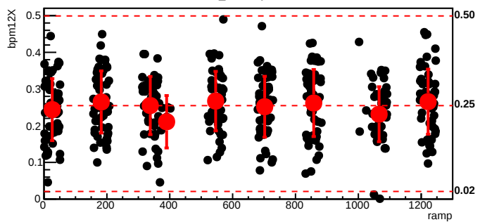
bmod_trim4,cyc=7804
