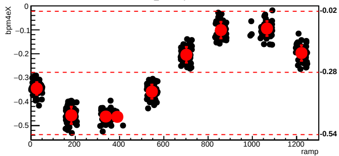
bmod_trim1,cyc=7804
