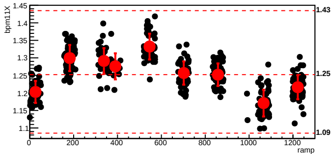
bmod_trim5,cyc=7828
