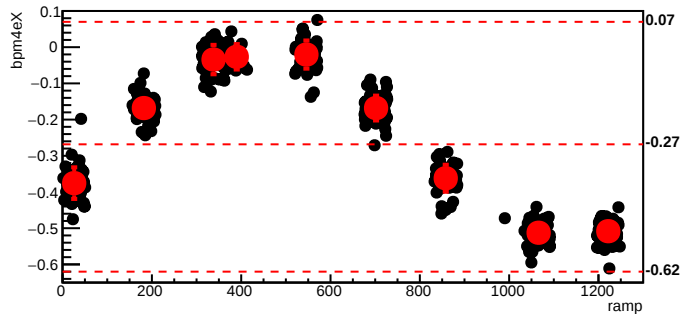
bmod_trim5,cyc=7828
