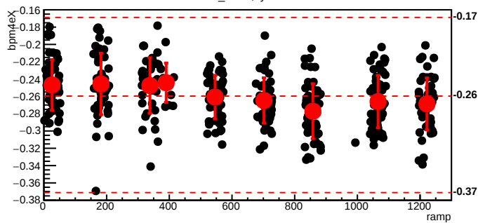
bmod_trim7,cyc=7828
