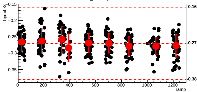
bmod_trim2,cyc=7828
