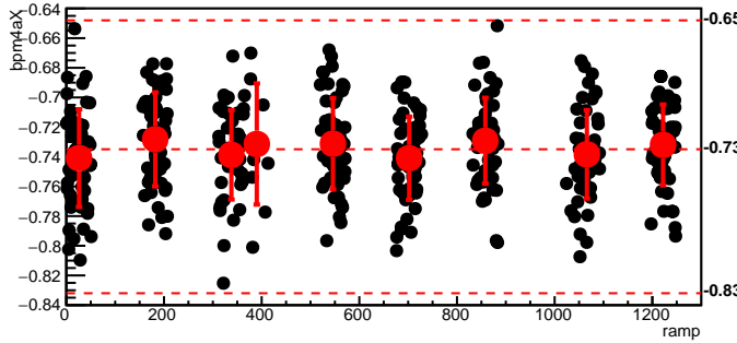
bmod_trim6,cyc=7865
