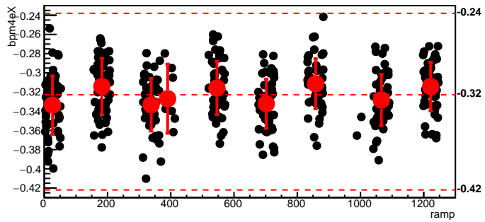
bmod_trim6,cyc=7865
