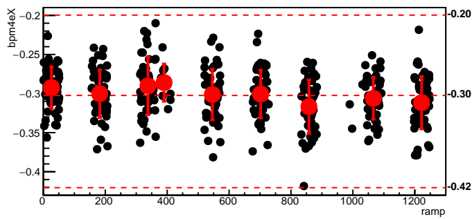
bmod_trim7,cyc=7865
