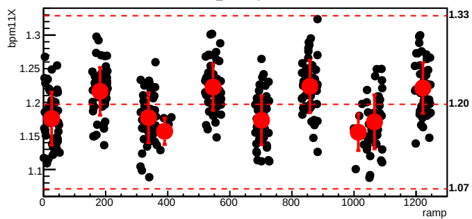
bmod_trim4,cyc=7873
