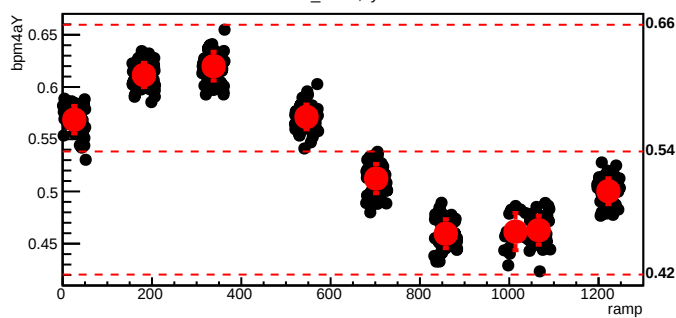
bmod_trim2,cyc=7873
