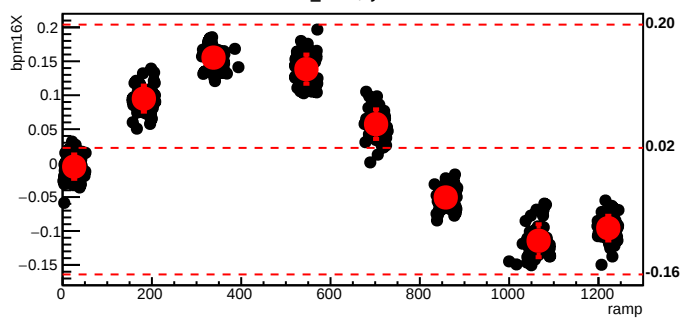
bmod_trim3,cyc=7873
