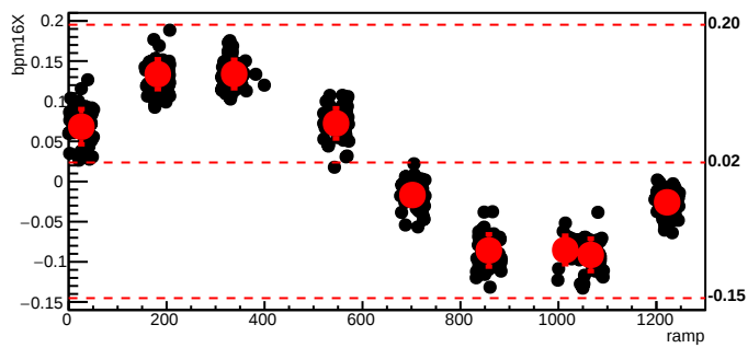
bmod_trim1,cyc=7873
