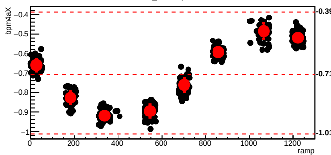
bmod_trim3,cyc=7873
