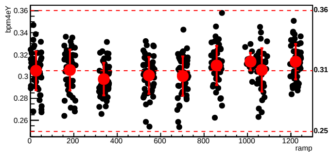
bmod_trim5,cyc=7873
