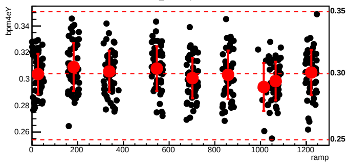
bmod_trim1,cyc=7873
