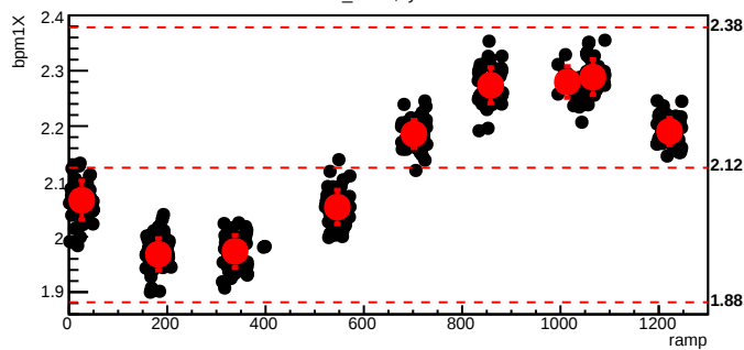
bmod_trim1,cyc=7873
