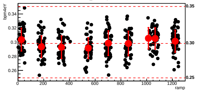
bmod_trim5,cyc=7994
