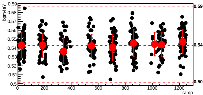
bmod_trim5,cyc=7994
