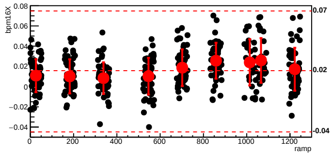
bmod_trim7,cyc=7994
