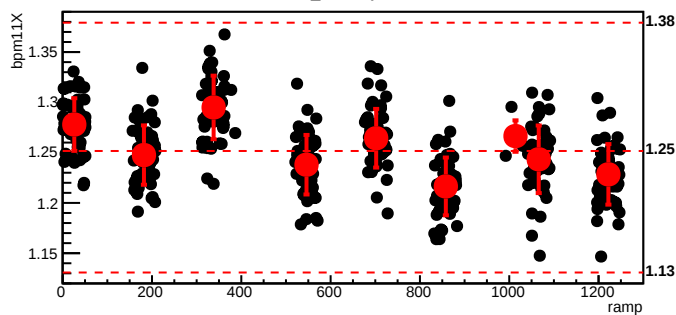
bmod_trim6,cyc=7994
