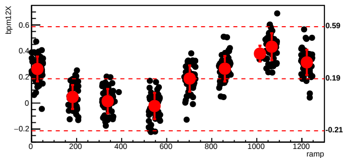
bmod_trim3,cyc=7994
