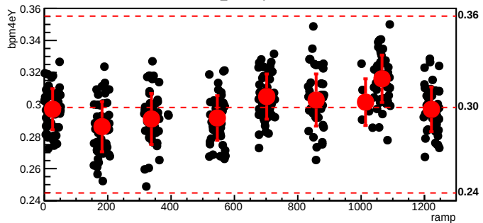
bmod_trim6,cyc=7994
