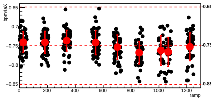
bmod_trim7,cyc=7994
