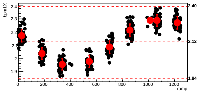
bmod_trim3,cyc=7994
