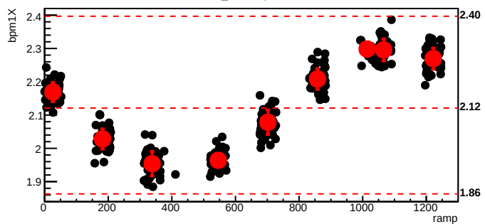
bmod_trim3,cyc=8020
