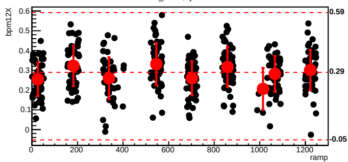
bmod_trim2,cyc=8020
