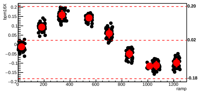
bmod_trim3,cyc=8020
