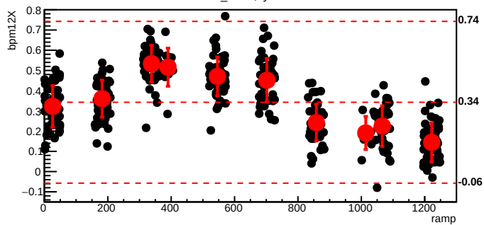
bmod_trim5,cyc=8020
