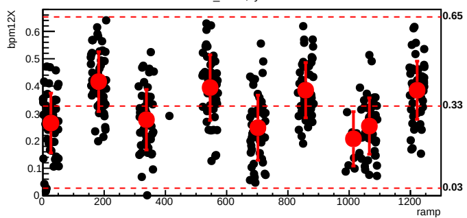
bmod_trim6,cyc=8020
