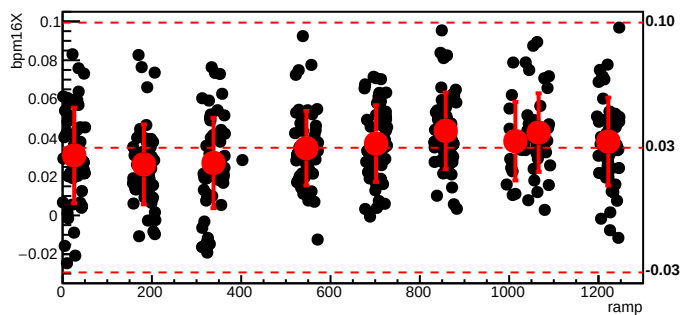
bmod_trim7,cyc=8020
