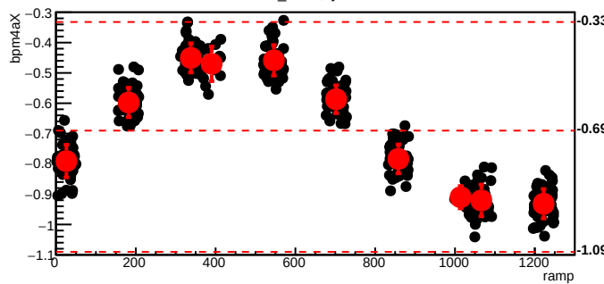
bmod_trim5,cyc=8020
