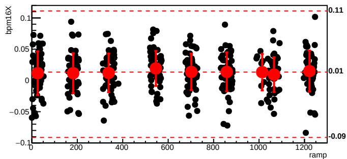
bmod_trim4,cyc=8020
