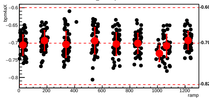
bmod_trim6,cyc=8020
