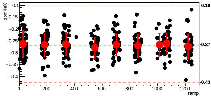
bmod_trim4,cyc=8020
