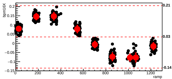
bmod_trim1,cyc=8020
