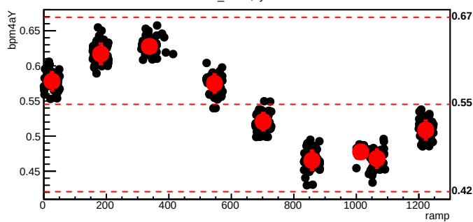
bmod_trim2,cyc=8020
