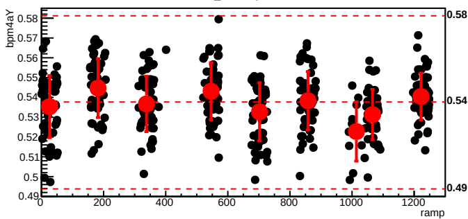
bmod_trim1,cyc=8020
