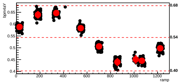
bmod_trim4,cyc=8020
