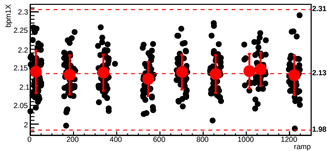
bmod_trim4,cyc=8020
