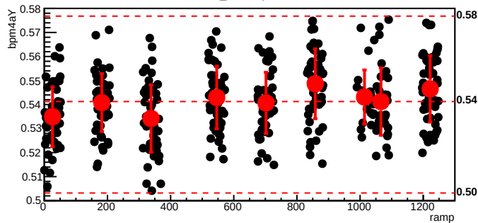
bmod_trim7,cyc=8020
