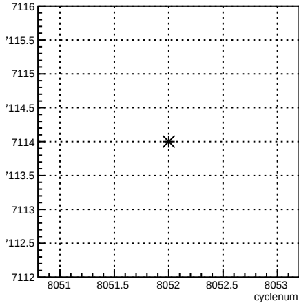
run:cyclenum {run == 7114}
