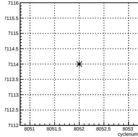
run:cyclenum {run == 7114}
