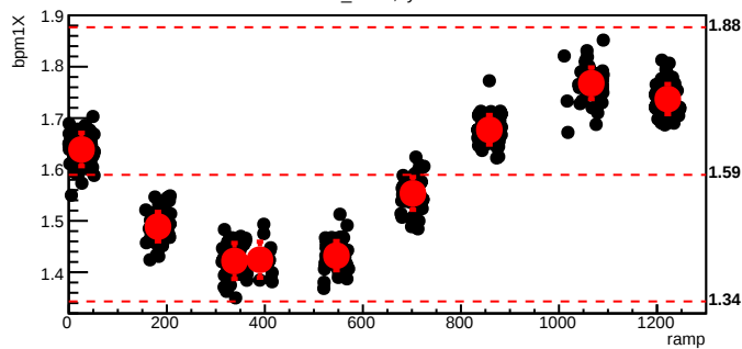
bmod_trim3,cyc=8052
