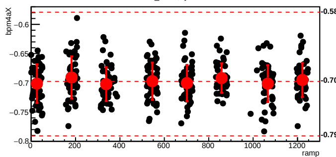
bmod_trim4,cyc=8052
