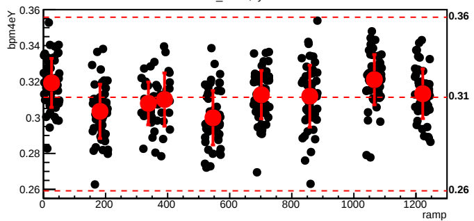
bmod_trim5,cyc=8052
