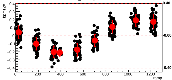
bmod_trim3,cyc=8052
