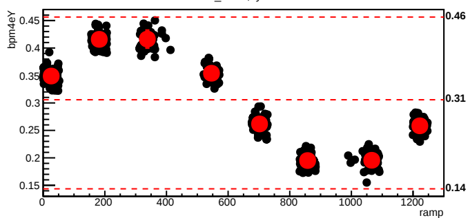
bmod_trim4,cyc=8052
