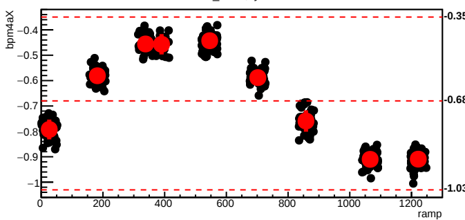
bmod_trim5,cyc=8052
