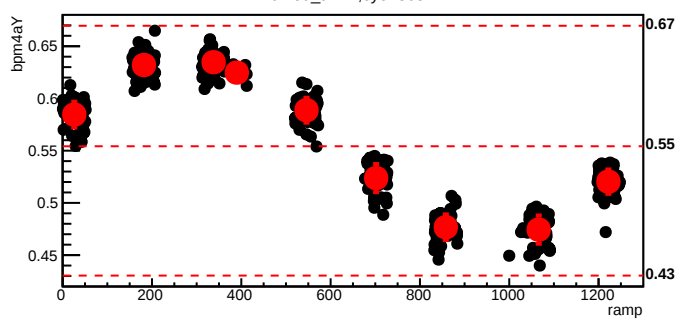
bmod_trim2,cyc=8052
