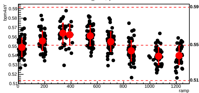
bmod_trim3,cyc=8052
