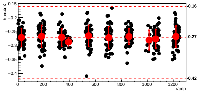
bmod_trim6,cyc=8052
