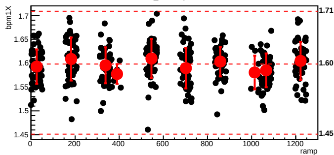
bmod_trim6,cyc=8052
