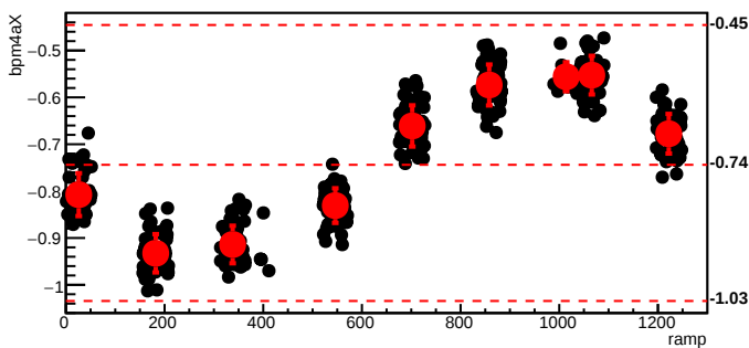
bmod_trim1,cyc=8052
