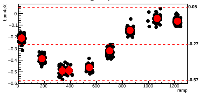
bmod_trim3,cyc=8052
