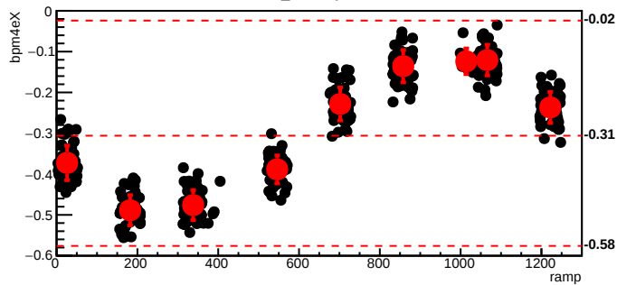
bmod_trim1,cyc=8052
