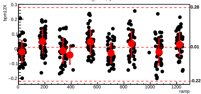
bmod_trim2,cyc=8052
