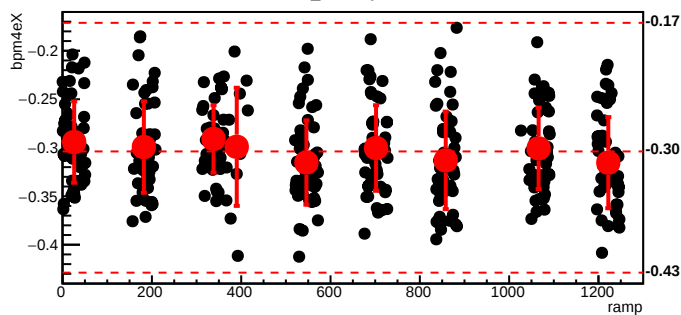
bmod_trim2,cyc=8054
