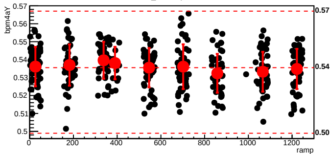
bmod_trim1,cyc=8054
