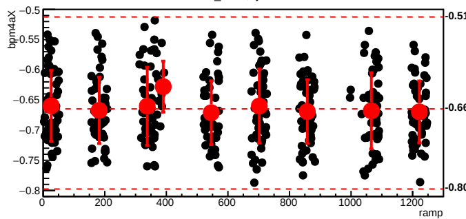
bmod_trim4,cyc=8065
