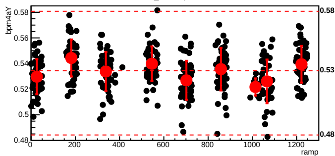
bmod_trim1,cyc=8065
