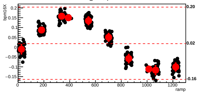
bmod_trim3,cyc=8065
