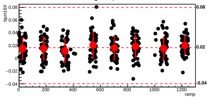
bmod_trim6,cyc=8065
