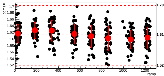
bmod_trim7,cyc=8065
