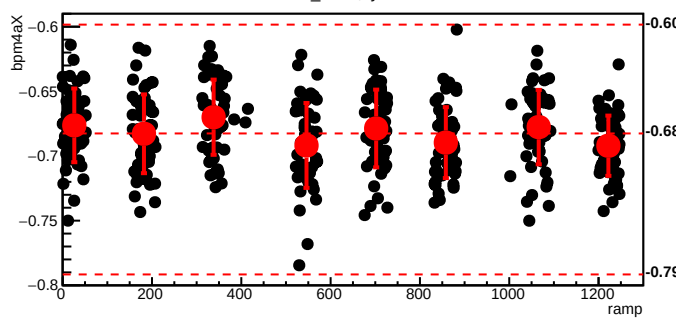
bmod_trim6,cyc=8065
