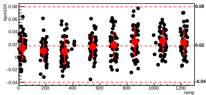
bmod_trim7,cyc=8065
