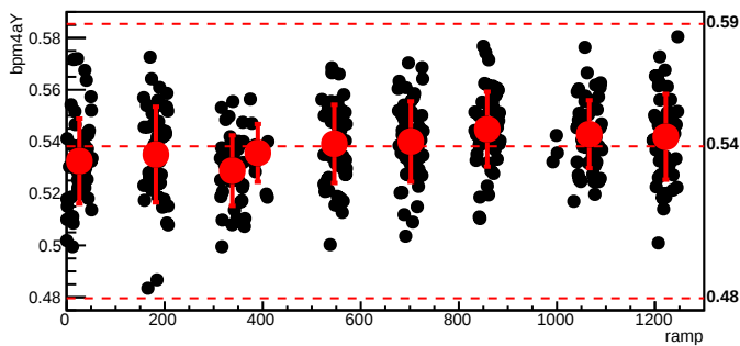
bmod_trim7,cyc=8145
