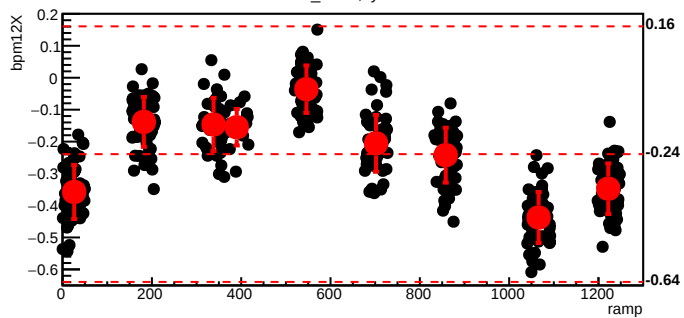
bmod_trim5,cyc=8145
