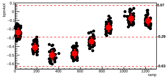
bmod_trim3,cyc=8145
