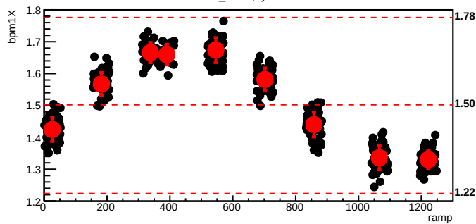
bmod_trim5,cyc=8145
