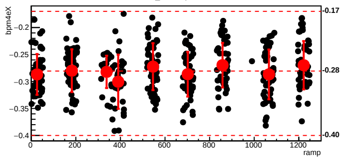
bmod_trim6,cyc=8263
