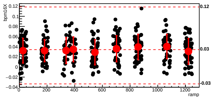
bmod_trim2,cyc=8263
