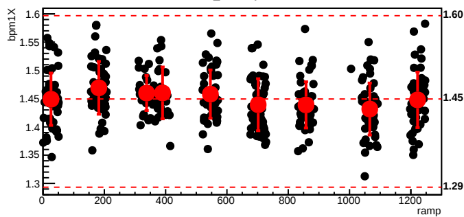
bmod_trim7,cyc=8263
