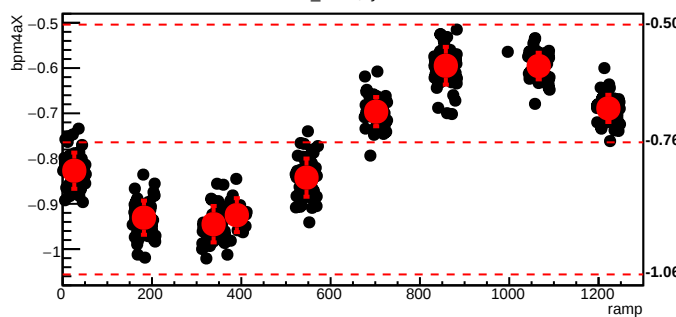
bmod_trim1,cyc=8263
