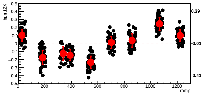
bmod_trim3,cyc=8263
