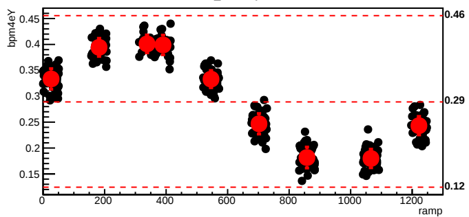
bmod_trim4,cyc=8263
