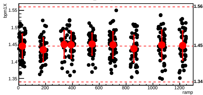
bmod_trim4,cyc=8263
