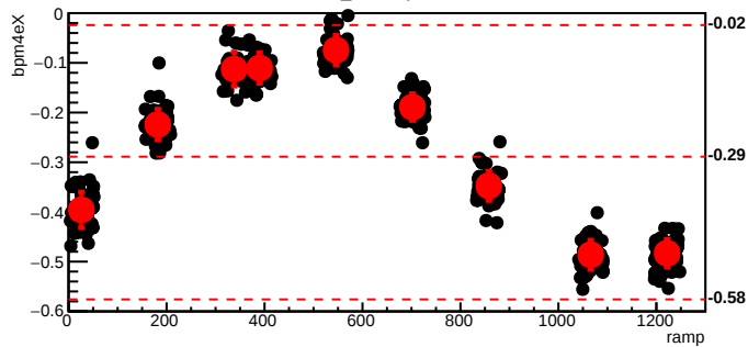
bmod_trim5,cyc=8263
