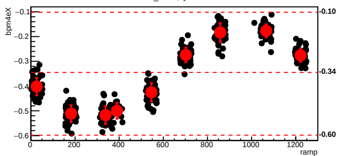
bmod_trim1,cyc=8263
