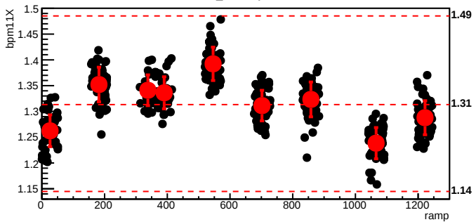
bmod_trim5,cyc=8263
