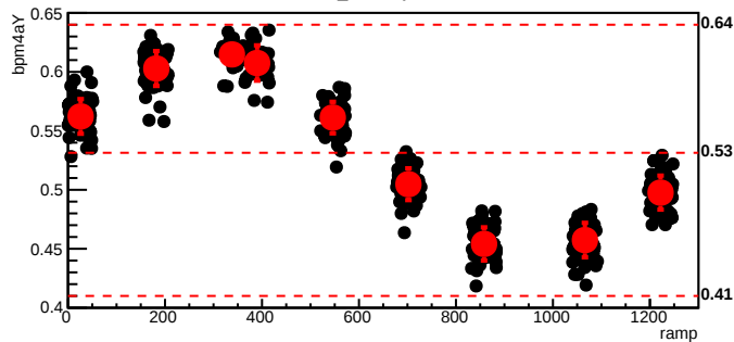
bmod_trim2,cyc=8263
