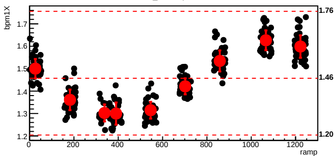
bmod_trim3,cyc=8263
