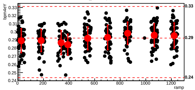
bmod_trim7,cyc=8263
