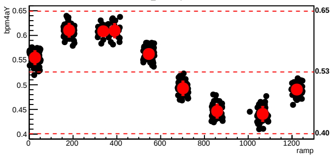
bmod_trim6,cyc=8263
