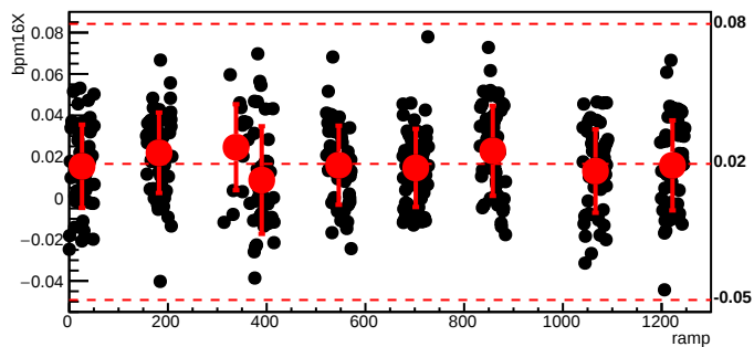
bmod_trim4,cyc=8279
