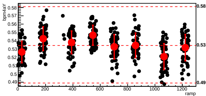
bmod_trim3,cyc=8279
