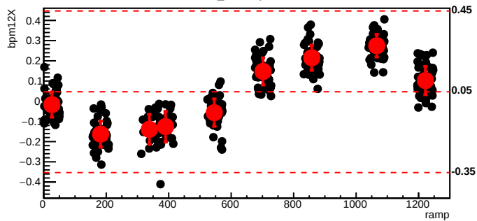
bmod_trim7,cyc=8279
