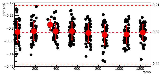
bmod_trim2,cyc=8279
