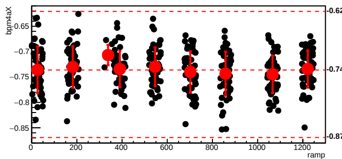
bmod_trim2,cyc=8279
