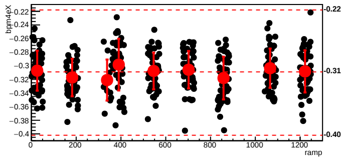
bmod_trim4,cyc=8279
