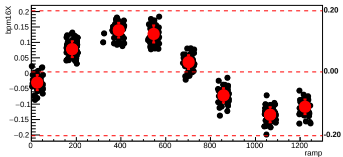
bmod_trim3,cyc=8279
