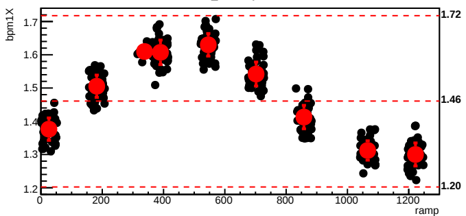
bmod_trim5,cyc=8279
