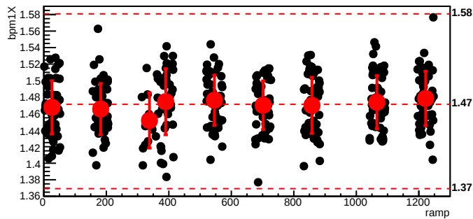
bmod_trim4,cyc=8279
