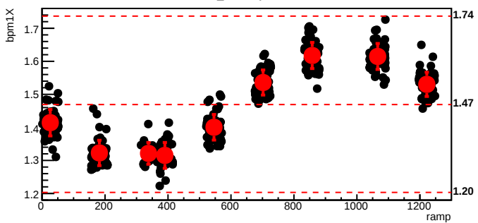
bmod_trim1,cyc=8279
