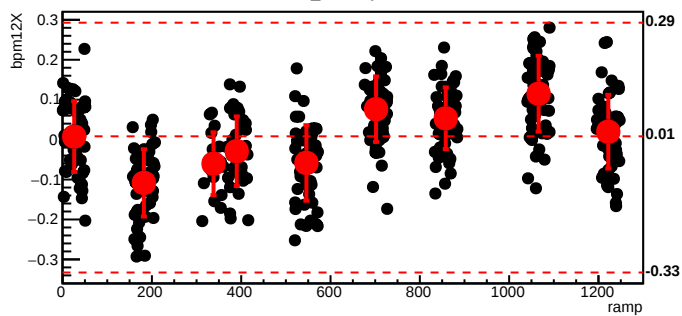
bmod_trim1,cyc=8279
