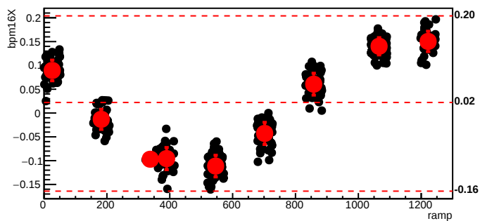
bmod_trim5,cyc=8279
