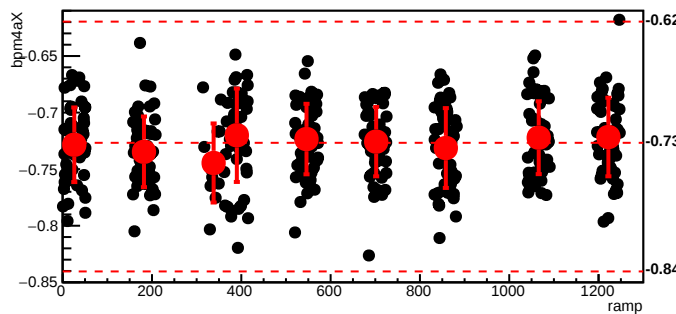
bmod_trim4,cyc=8279
