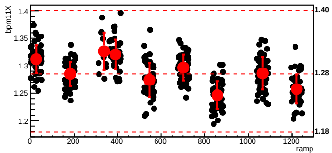
bmod_trim6,cyc=8279
