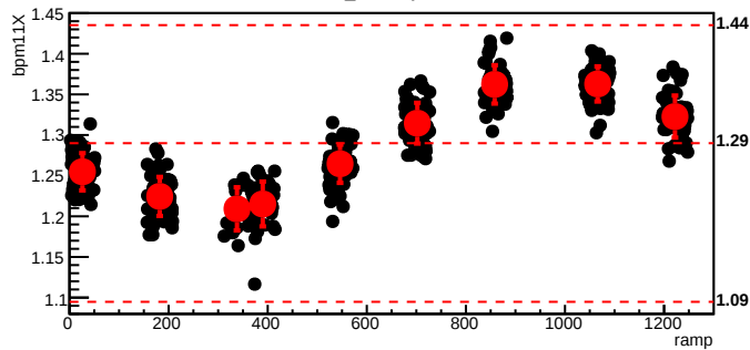
bmod_trim7,cyc=8279
