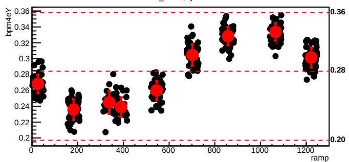
bmod_trim6,cyc=8322
