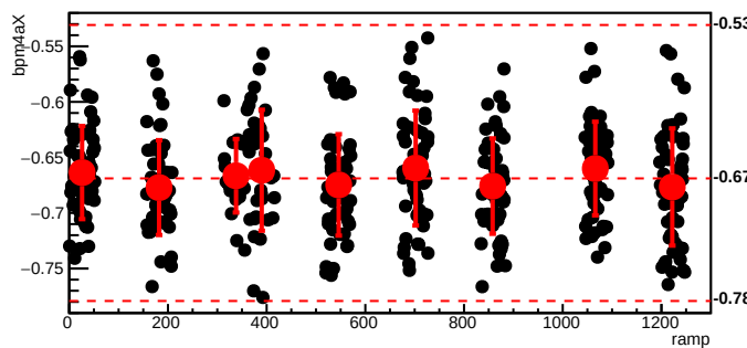
bmod_trim4,cyc=8322
