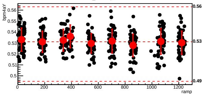
bmod_trim1,cyc=8322
