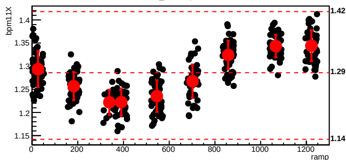
bmod_trim3,cyc=8322
