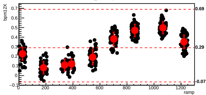
bmod_trim7,cyc=8322
