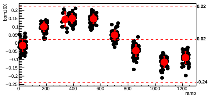
bmod_trim3,cyc=8322
