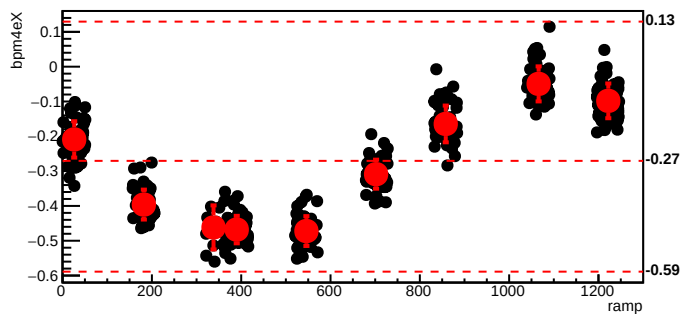
bmod_trim3,cyc=8322
