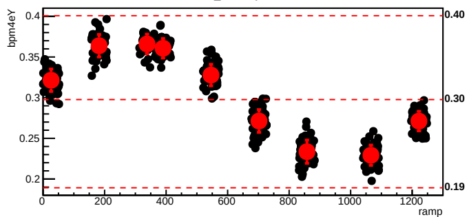
bmod_trim2,cyc=8322
