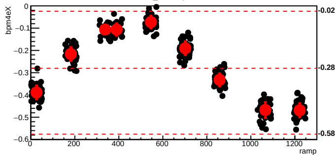
bmod_trim5,cyc=8322
