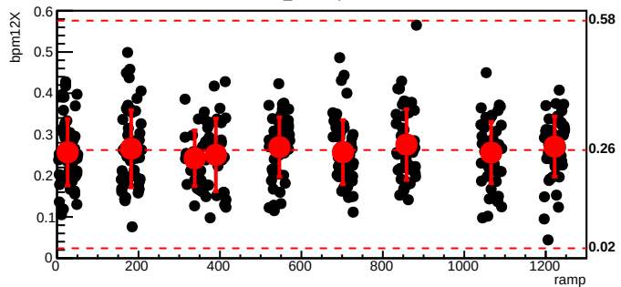
bmod_trim4,cyc=8322
