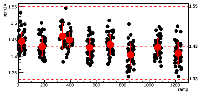
bmod_trim7,cyc=8322
