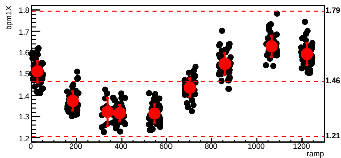
bmod_trim3,cyc=8322
