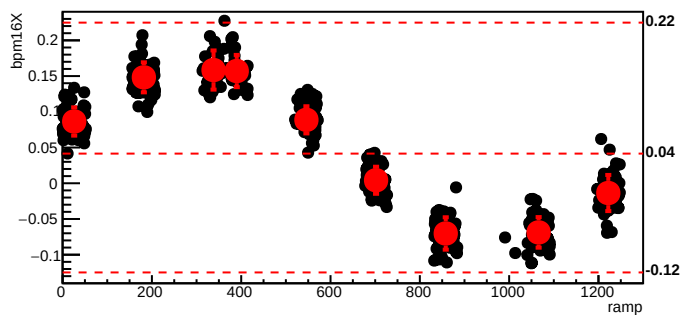
bmod_trim1,cyc=8322
