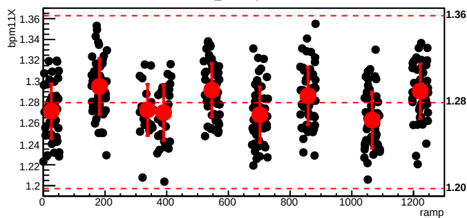
bmod_trim2,cyc=8322
