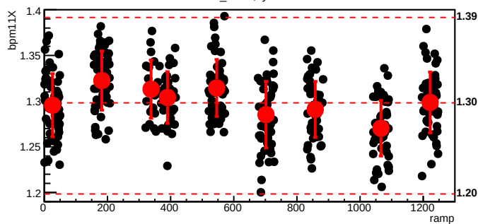
bmod_trim6,cyc=8322
