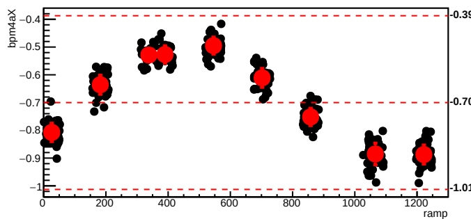
bmod_trim5,cyc=8322
