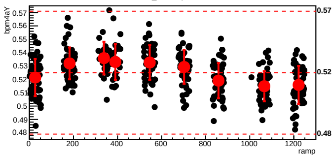
bmod_trim3,cyc=8319
