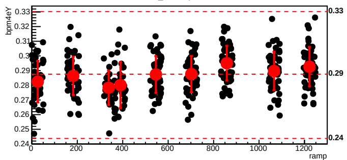
bmod_trim7,cyc=8319
