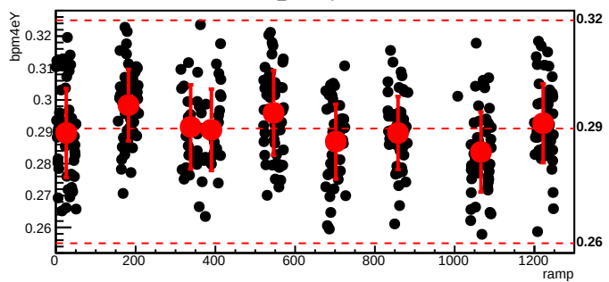
bmod_trim1,cyc=8319
