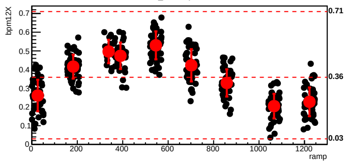
bmod_trim5,cyc=8319
