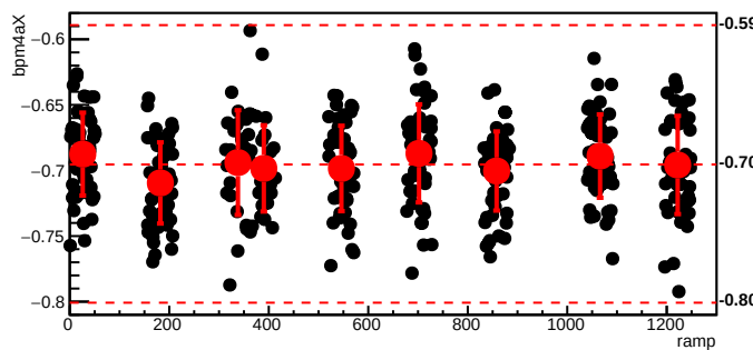
bmod_trim6,cyc=8319
