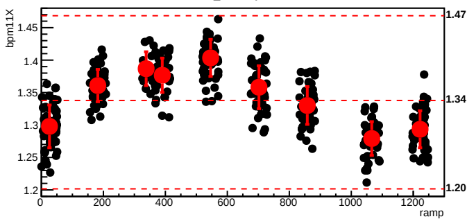
bmod_trim5,cyc=8319
