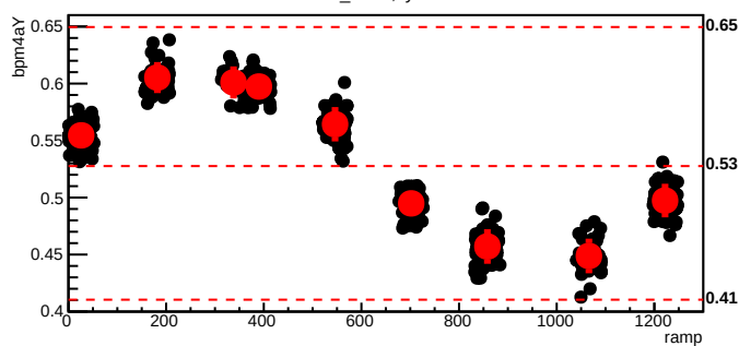
bmod_trim2,cyc=8319
