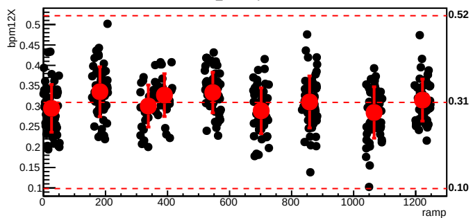
bmod_trim6,cyc=8319
