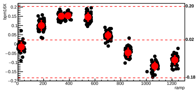
bmod_trim3,cyc=8319
