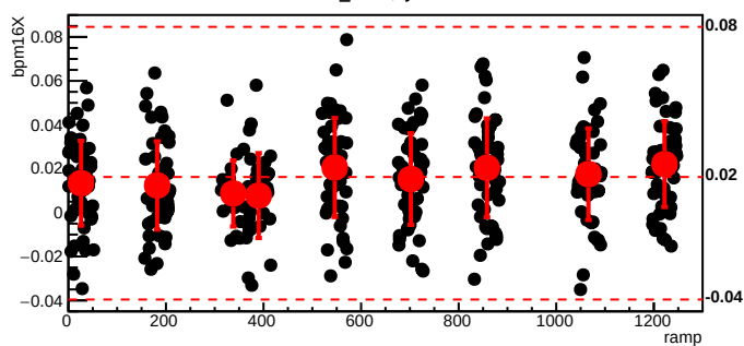
bmod_trim2,cyc=8319
