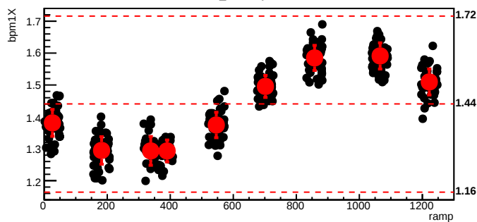
bmod_trim1,cyc=8327
