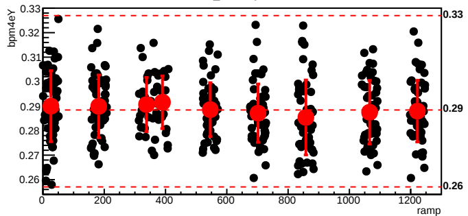
bmod_trim1,cyc=8327
