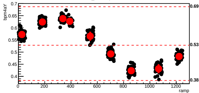
bmod_trim4,cyc=8328
