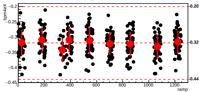
bmod_trim2,cyc=8328
