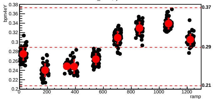
bmod_trim6,cyc=8328
