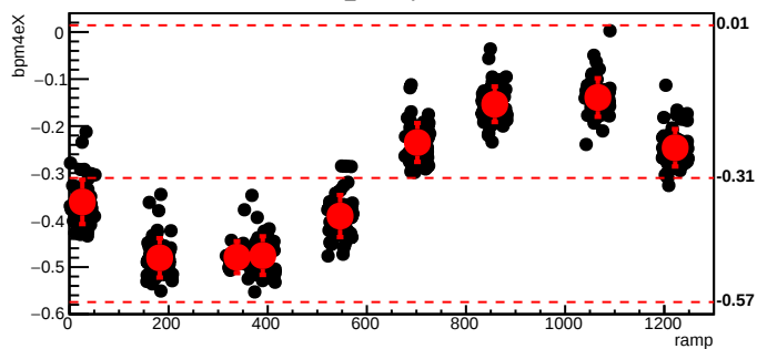
bmod_trim1,cyc=8328
