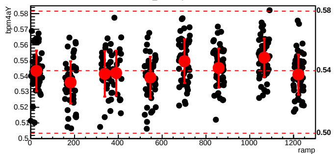
bmod_trim7,cyc=8328
