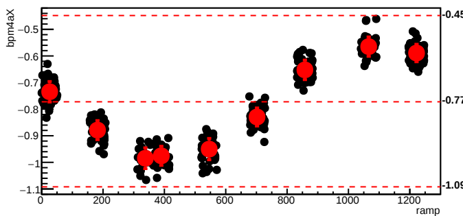
bmod_trim3,cyc=8328
