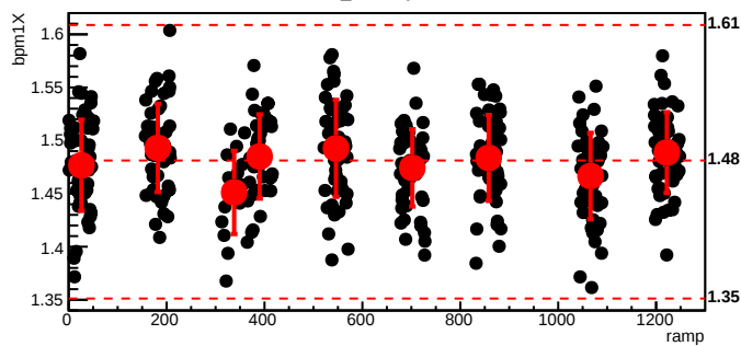
bmod_trim2,cyc=8328
