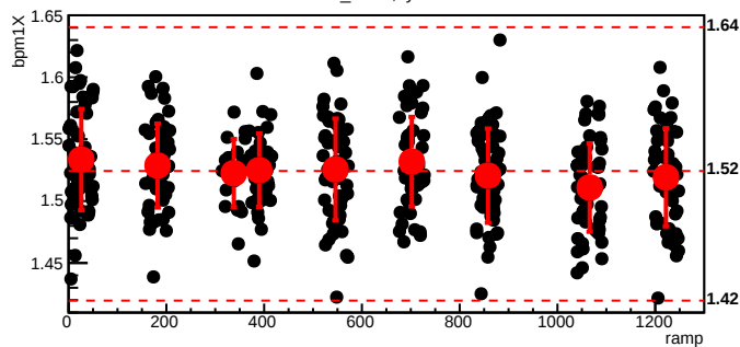
bmod_trim6,cyc=8328
