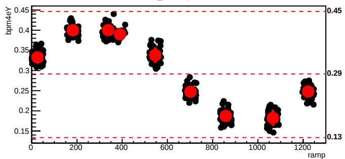
bmod_trim4,cyc=8328
