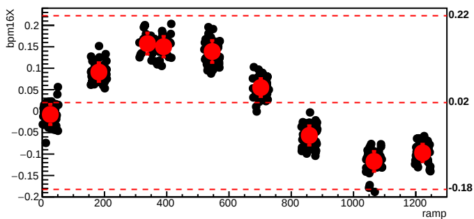
bmod_trim3,cyc=8328
