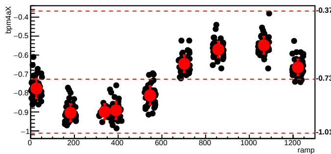
bmod_trim1,cyc=8328
