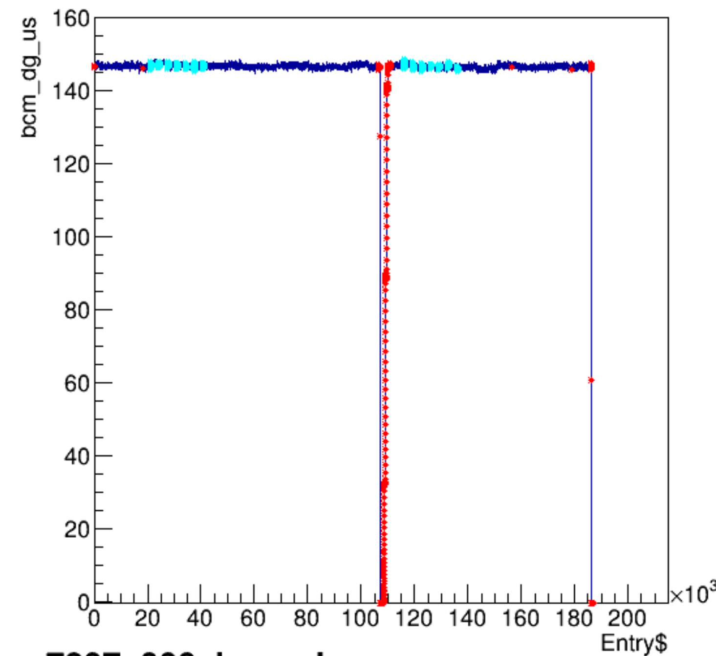
bcm_dg_us:Entry$
