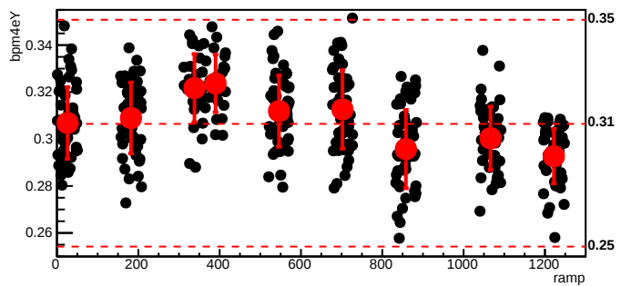
bmod_trim3,cyc=8379
