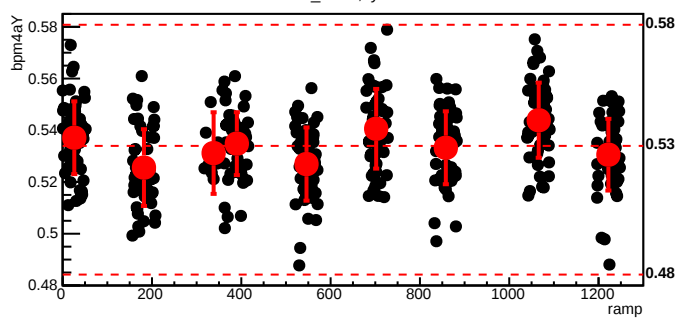
bmod_trim7,cyc=8379
