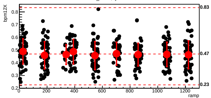
bmod_trim4,cyc=8379
