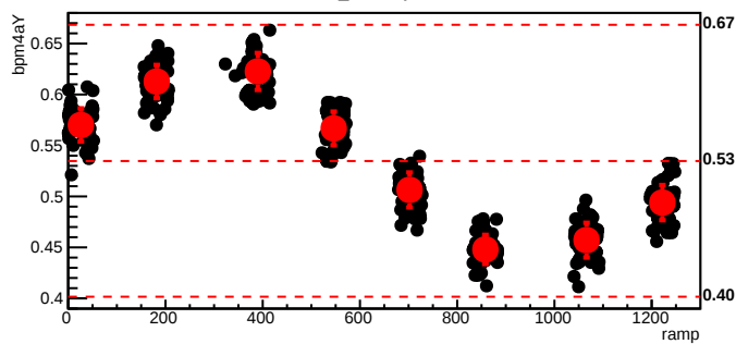
bmod_trim6,cyc=8379
