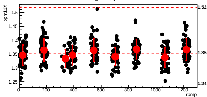
bmod_trim4,cyc=8379
