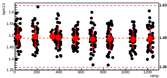
bmod_trim2,cyc=8379
