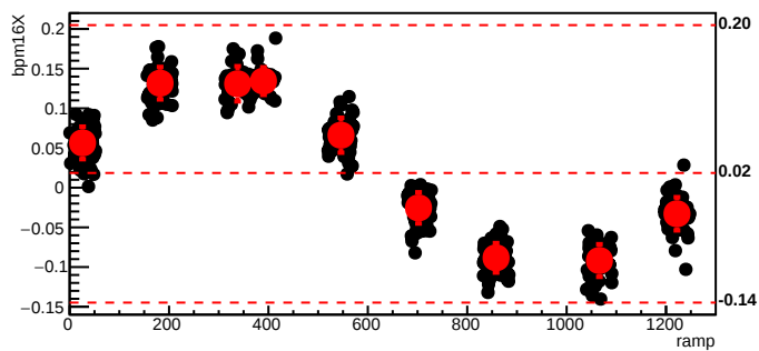
bmod_trim1,cyc=8379
