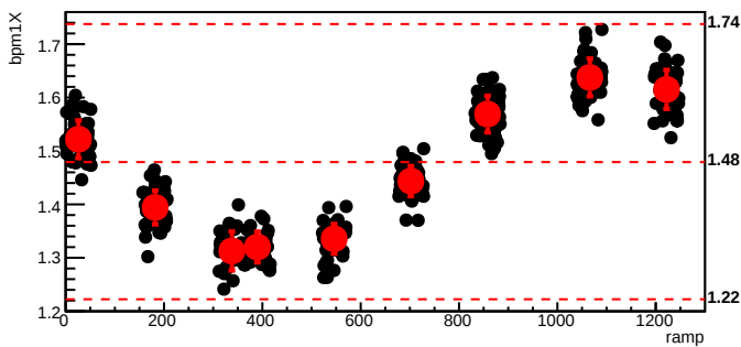
bmod_trim3,cyc=8379
