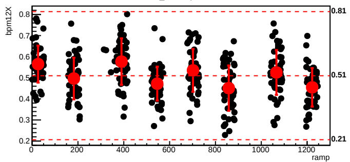
bmod_trim6,cyc=8379
