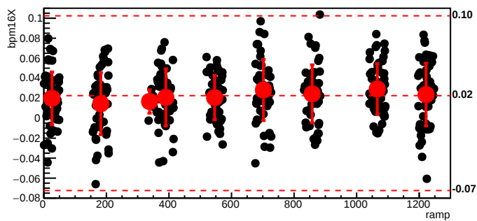
bmod_trim2,cyc=8379
