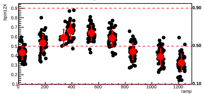
bmod_trim5,cyc=8379
