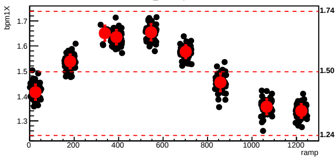
bmod_trim5,cyc=8379
