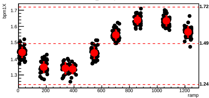
bmod_trim1,cyc=8379
