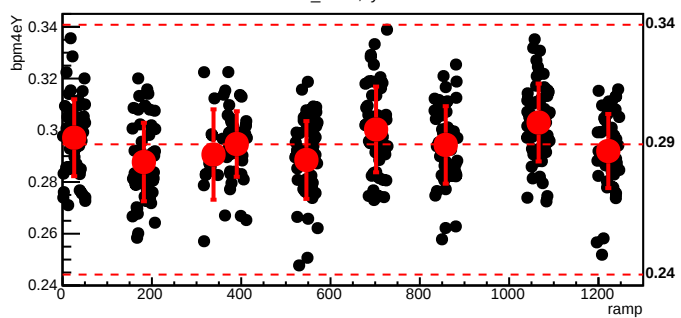
bmod_trim7,cyc=8379
