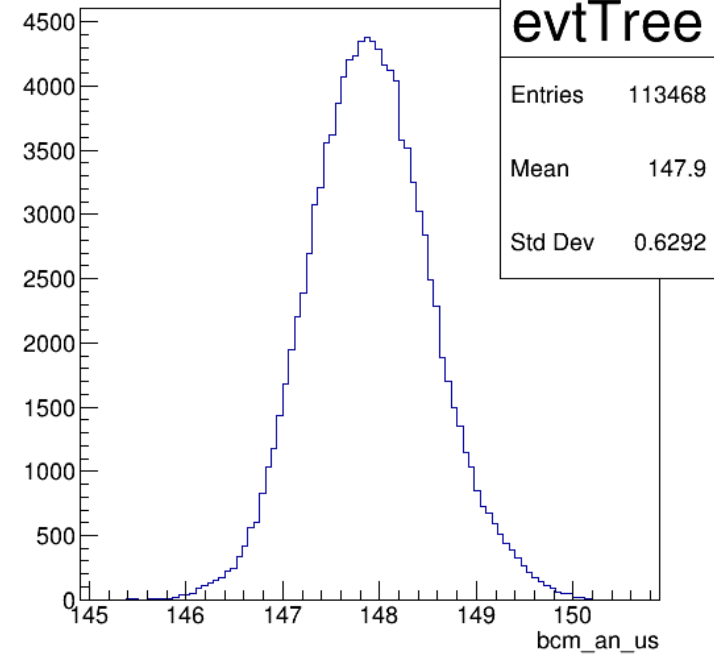
bcm_an_us {ErrorFlag==0}
