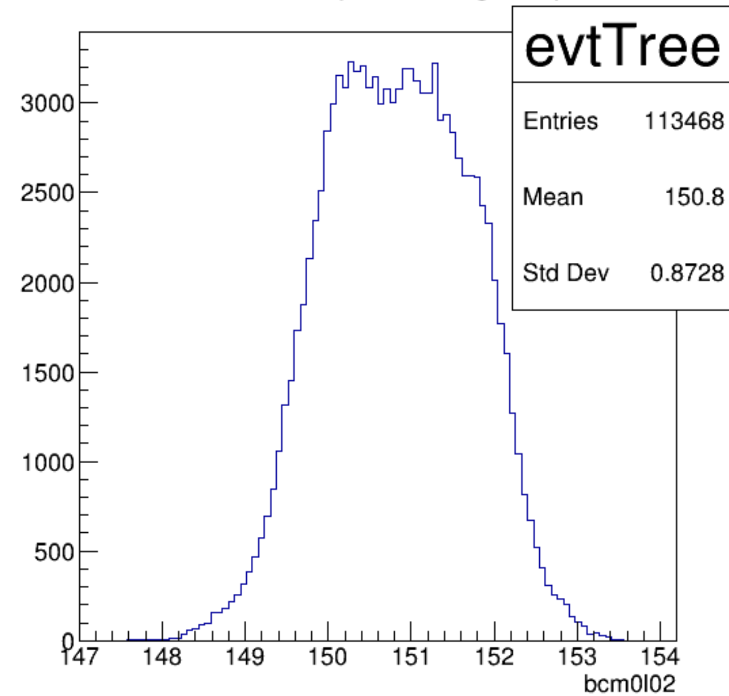
bcm0l02 {ErrorFlag==0}
