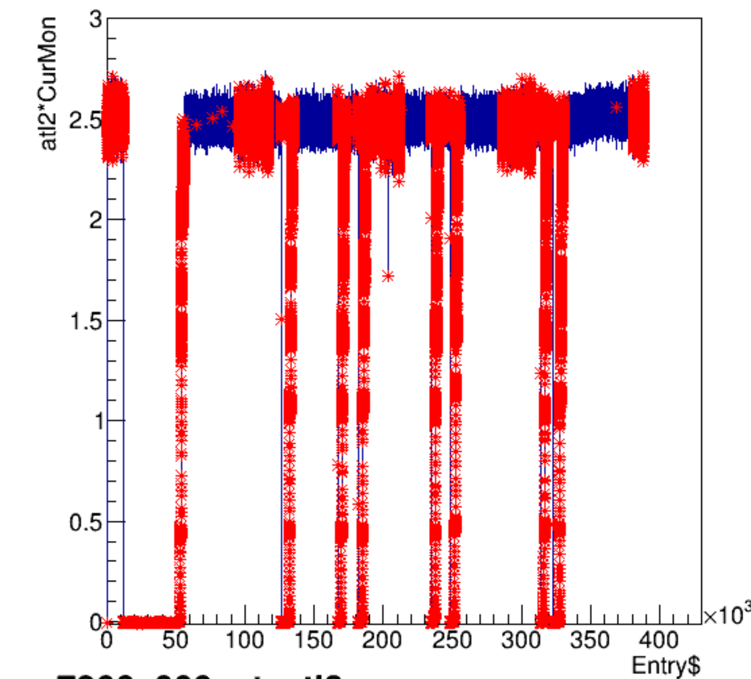
atl2*CurMon:Entry$
