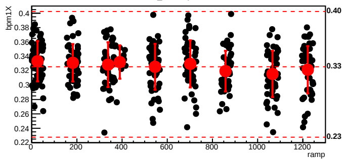
bmod_trim2,cyc=8559
