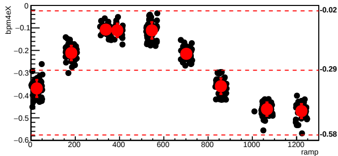
bmod_trim7,cyc=8559
