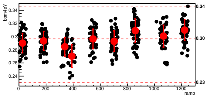
bmod_trim7,cyc=8559
