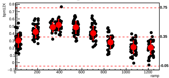
bmod_trim6,cyc=8559
