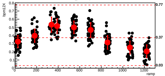
bmod_trim5,cyc=8559
