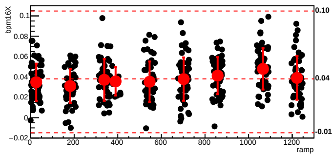
bmod_trim2,cyc=8559
