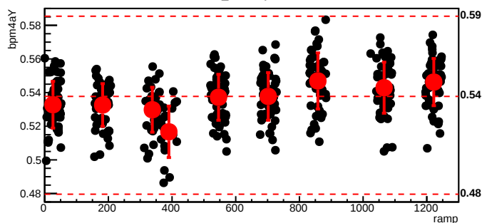
bmod_trim7,cyc=8559
