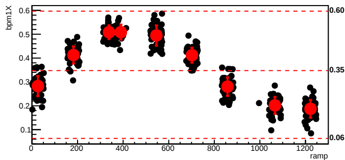
bmod_trim7,cyc=8559
