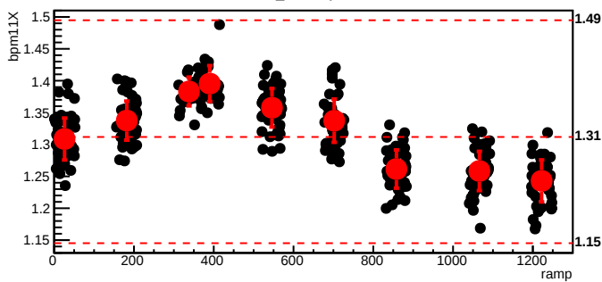
bmod_trim6,cyc=8559
