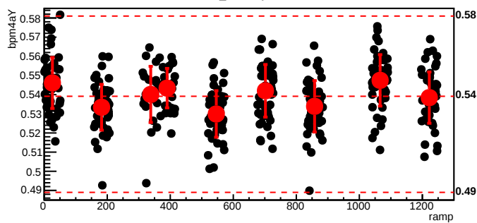
bmod_trim5,cyc=8559
