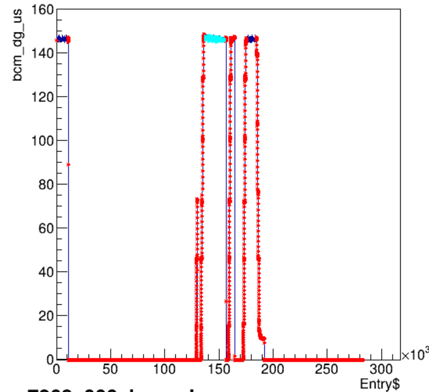
bcm_dg_us:Entry$
