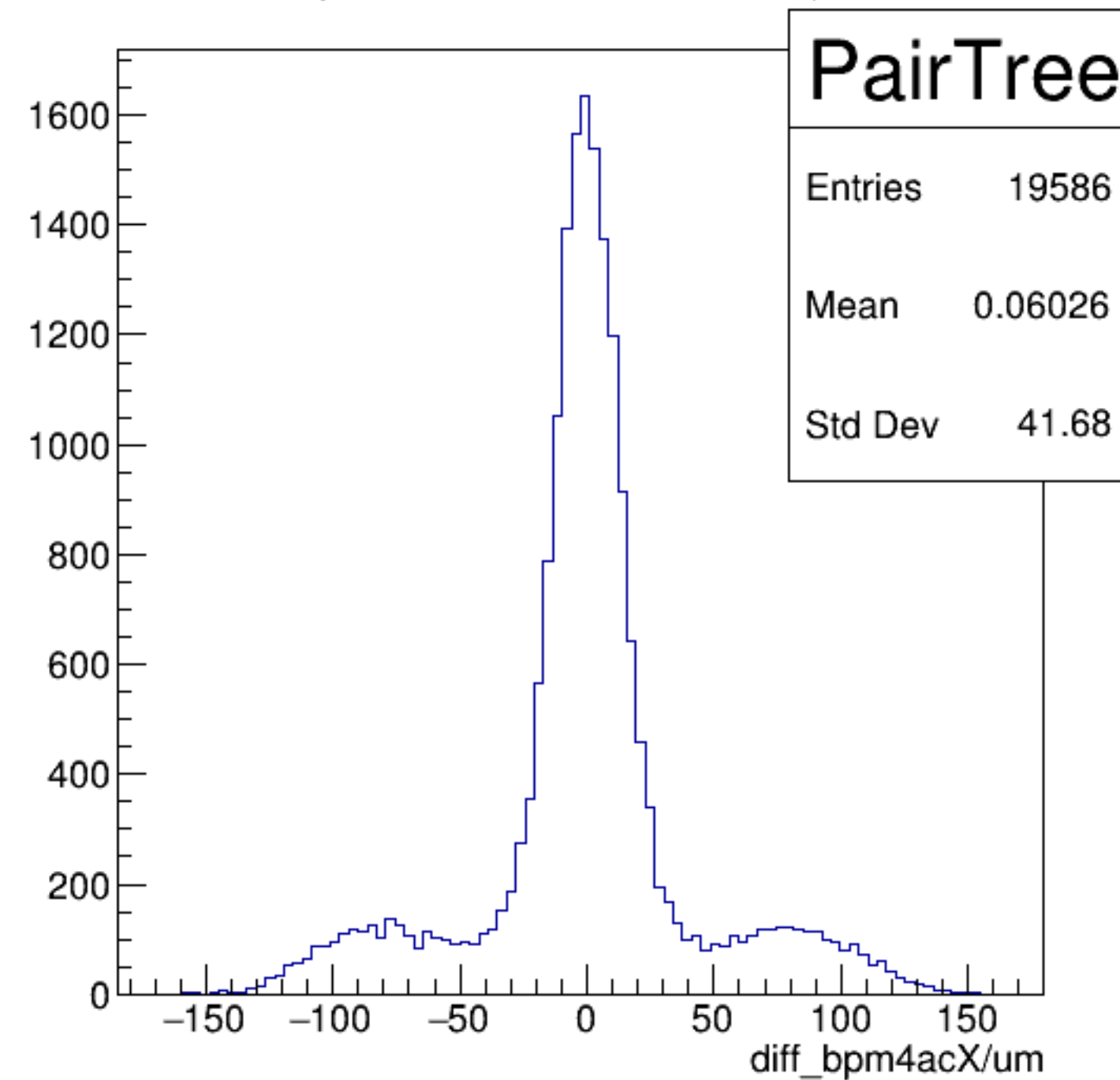
diff_bpm4acX/um {ErrorFlag==0}
