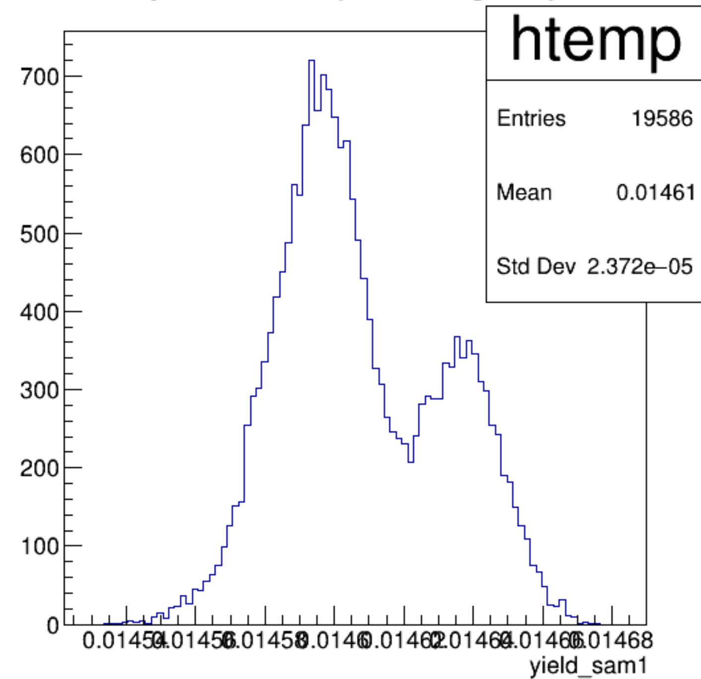
yield_sam1 {ErrorFlag==0}
