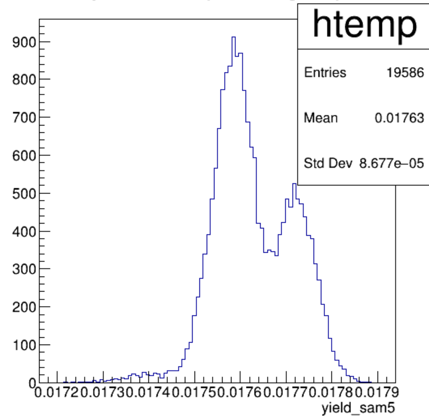
yield_sam5 {ErrorFlag==0}
