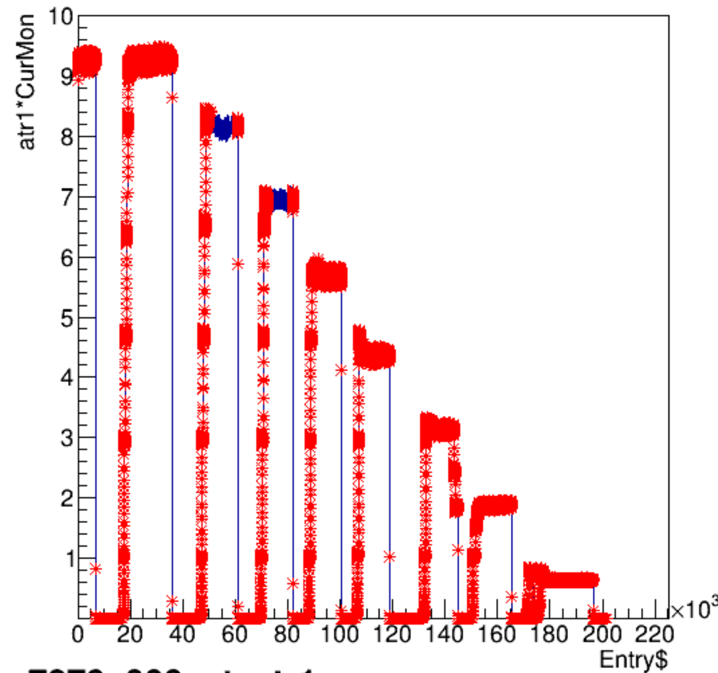
atr1*CurMon:Entry$
