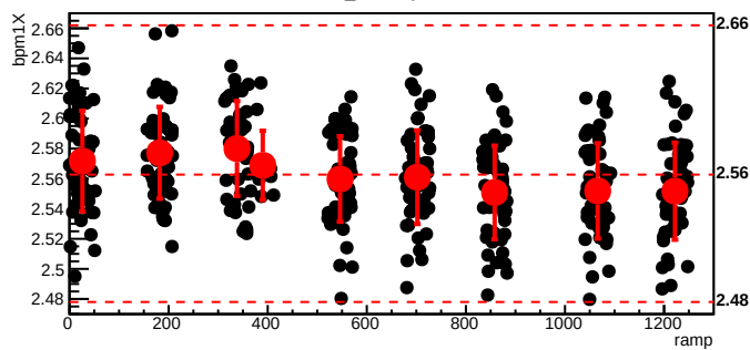
bmod_trim7,cyc=8569
