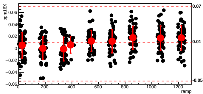
bmod_trim7,cyc=8569
