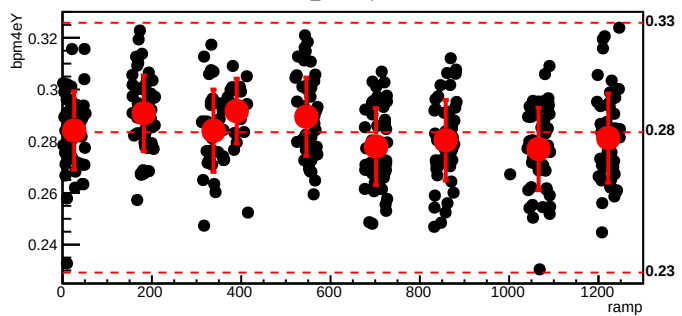
bmod_trim1,cyc=8569
