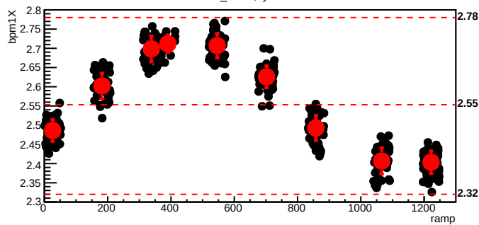
bmod_trim5,cyc=8569
