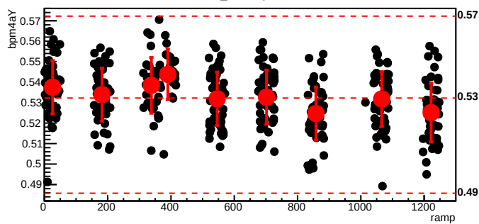
bmod_trim1,cyc=8569
