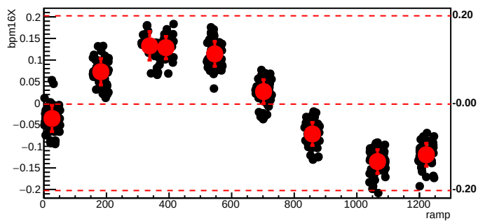
bmod_trim3,cyc=8569
