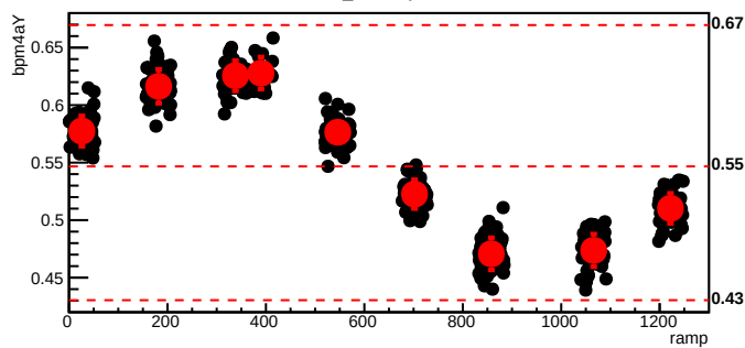
bmod_trim2,cyc=8569
