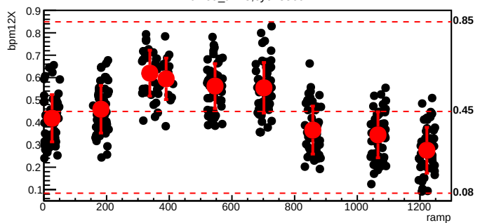
bmod_trim5,cyc=8569
