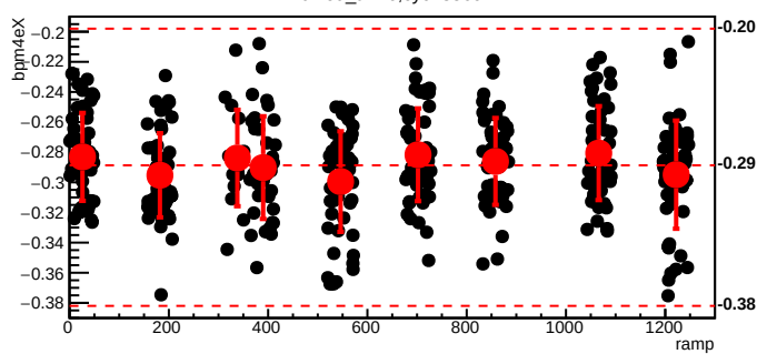
bmod_trim6,cyc=8569
