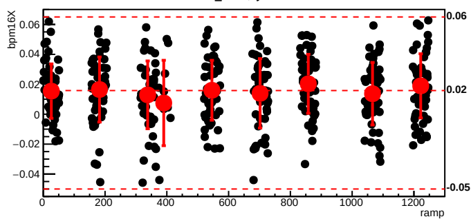
bmod_trim4,cyc=8569
