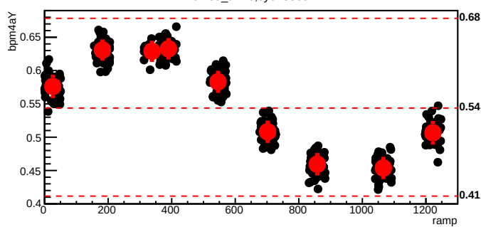
bmod_trim6,cyc=8569
