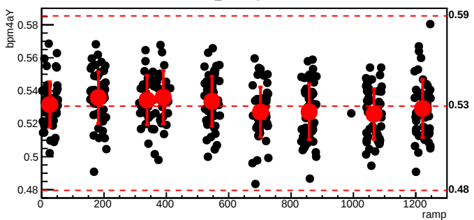
bmod_trim1,cyc=8574
