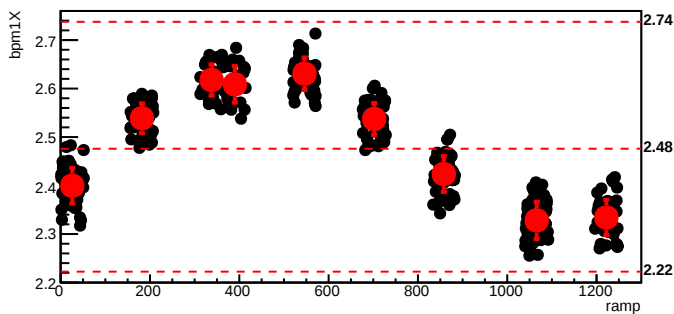
bmod_trim5,cyc=8574
