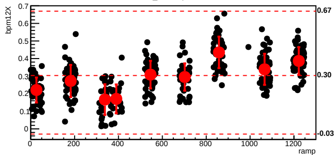
bmod_trim1,cyc=8574
