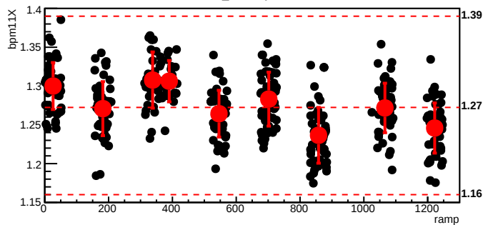
bmod_trim6,cyc=8574
