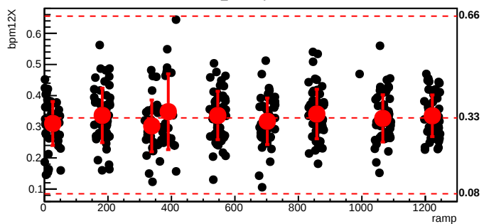
bmod_trim4,cyc=8574
