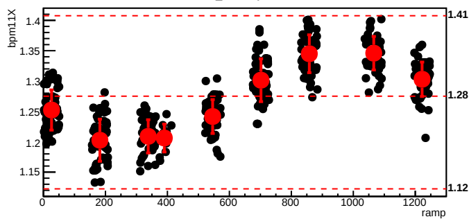
bmod_trim7,cyc=8574
