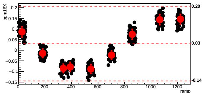
bmod_trim5,cyc=8574
