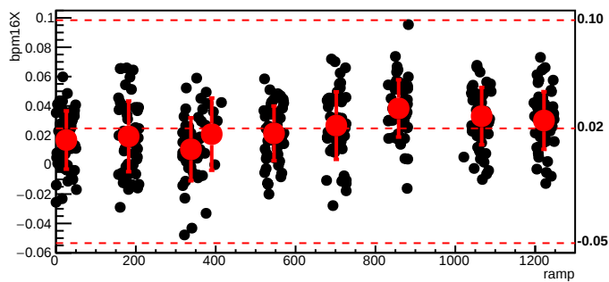
bmod_trim7,cyc=8574
