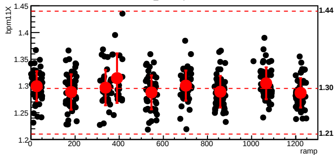
bmod_trim4,cyc=8574
