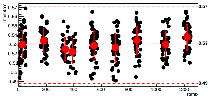
bmod_trim5,cyc=8574
