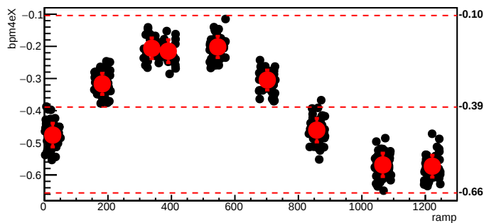
bmod_trim5,cyc=8574
