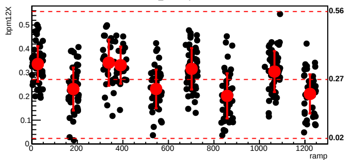
bmod_trim6,cyc=8574
