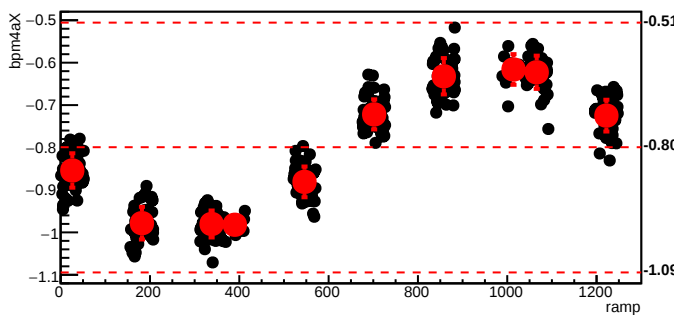
bmod_trim1,cyc=8584
