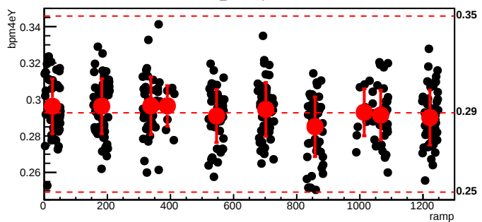
bmod_trim1,cyc=8584
