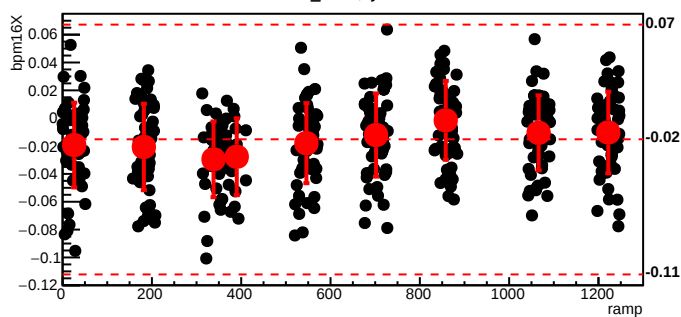
bmod_trim7,cyc=8584
