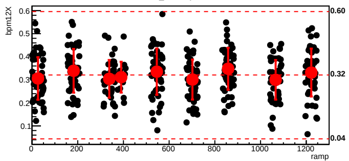
bmod_trim4,cyc=8584
