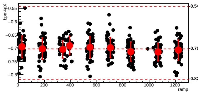
bmod_trim2,cyc=8584
