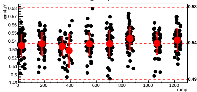
bmod_trim7,cyc=8584
