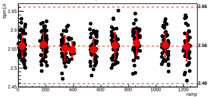
bmod_trim4,cyc=8584
