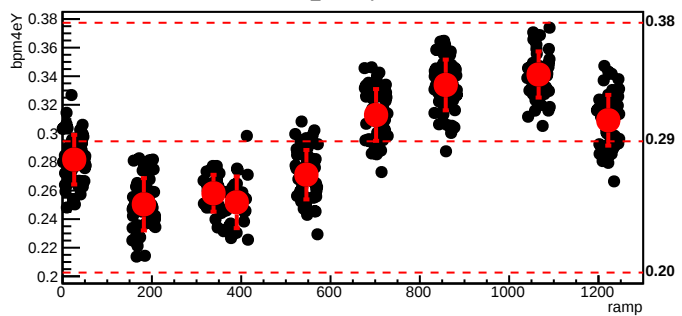
bmod_trim6,cyc=8584
