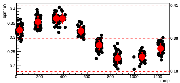
bmod_trim2,cyc=8584
