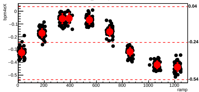
bmod_trim5,cyc=8584
