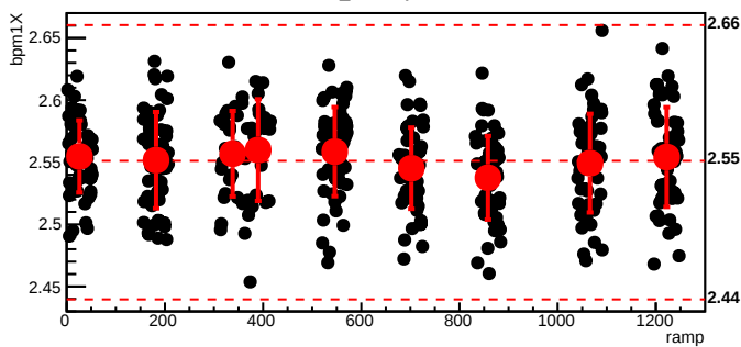
bmod_trim6,cyc=8584
