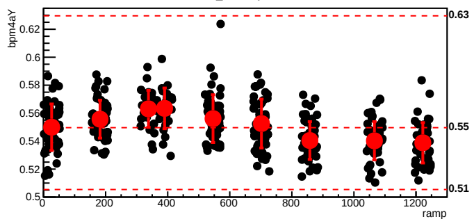
bmod_trim3,cyc=8584
