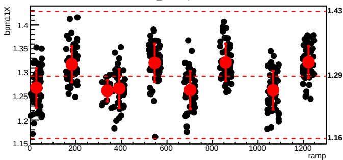
bmod_trim4,cyc=8590
