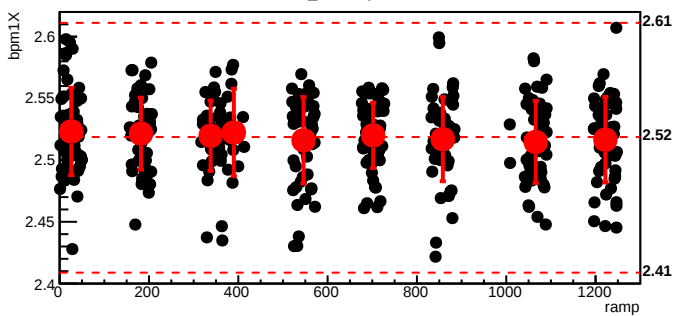
bmod_trim2,cyc=8590
