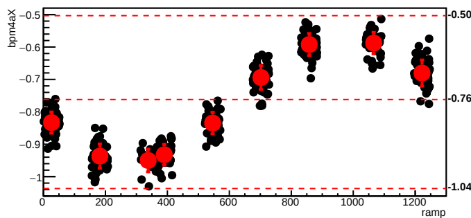
bmod_trim1,cyc=8590
