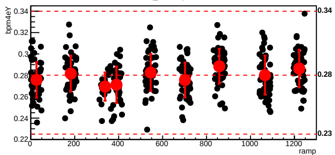
bmod_trim7,cyc=8590
