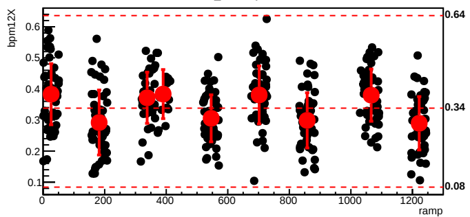
bmod_trim2,cyc=8590
