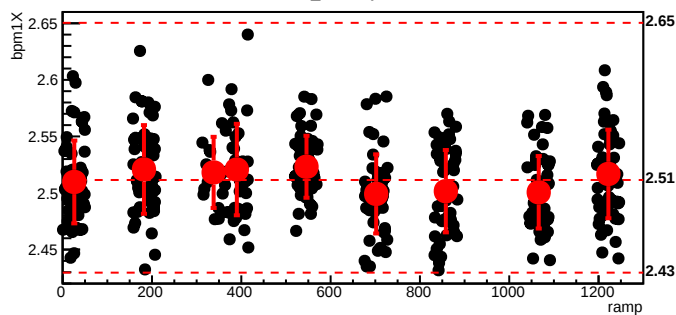
bmod_trim7,cyc=8590
