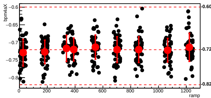
bmod_trim6,cyc=8590
