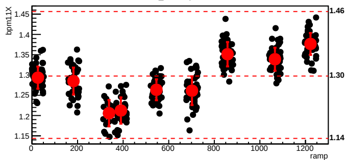
bmod_trim3,cyc=8590
