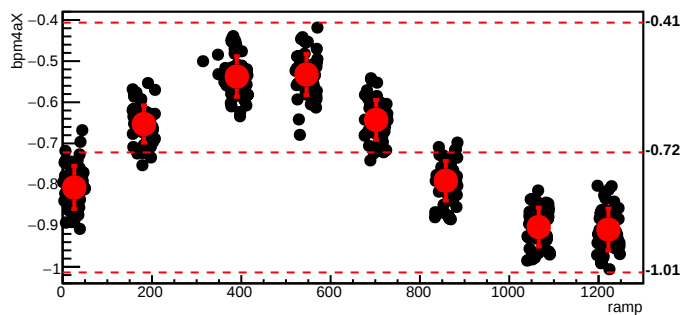
bmod_trim5,cyc=8590
