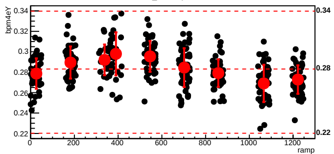
bmod_trim3,cyc=8590
