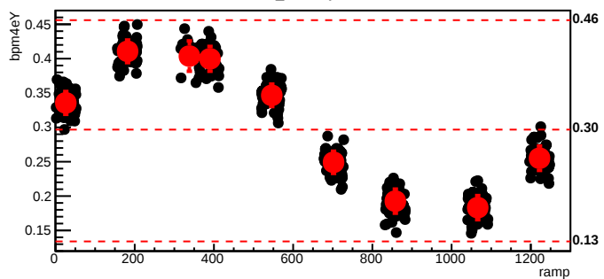
bmod_trim4,cyc=8590
