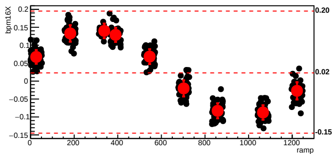
bmod_trim1,cyc=8590
