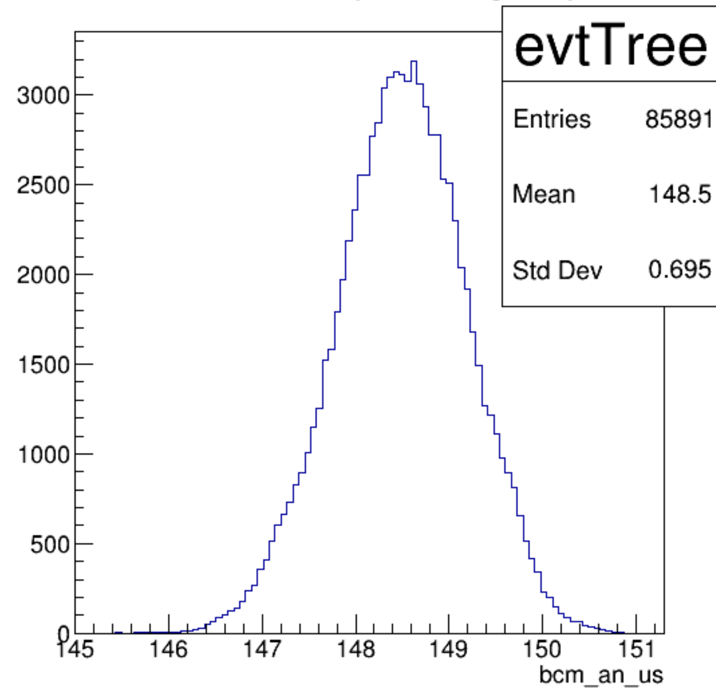
bcm_an_us {ErrorFlag==0}
