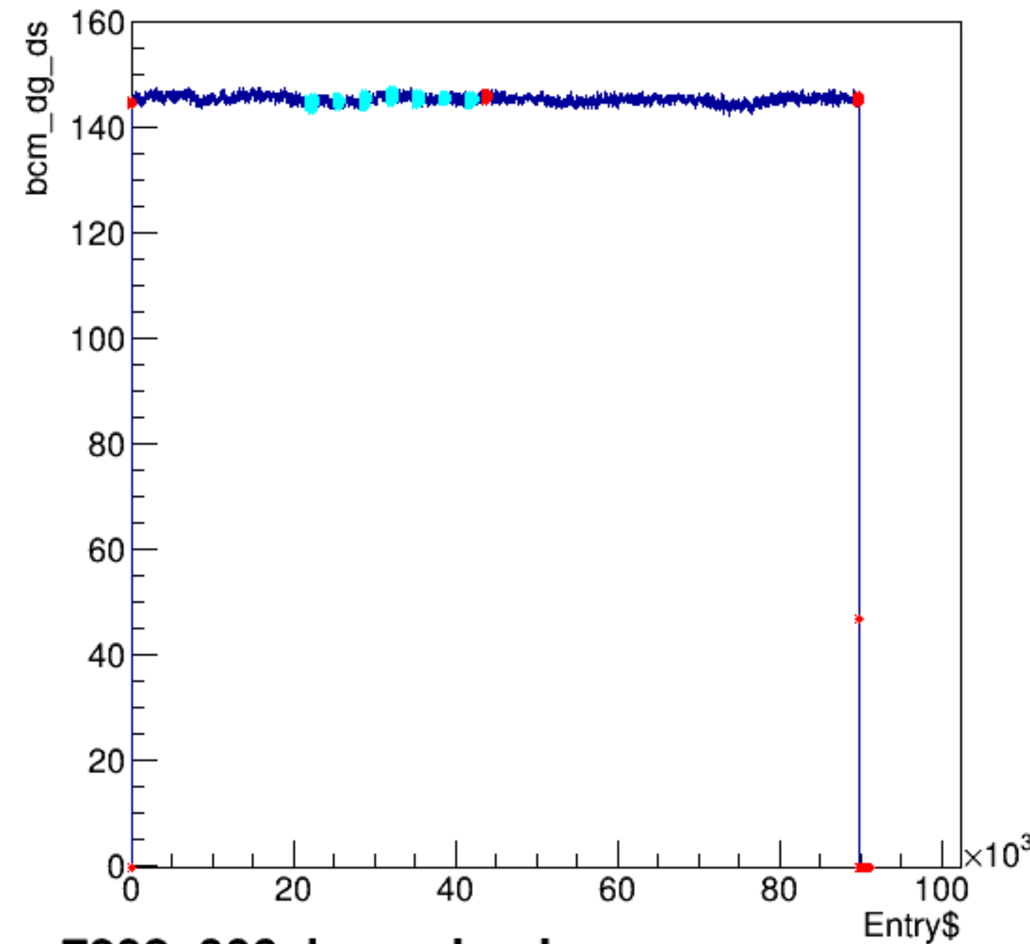
bcm_dg_ds:Entry$
