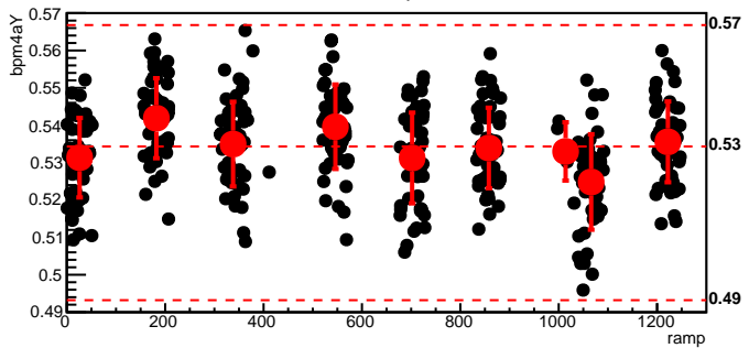
bmod_trim1,cyc=8599
