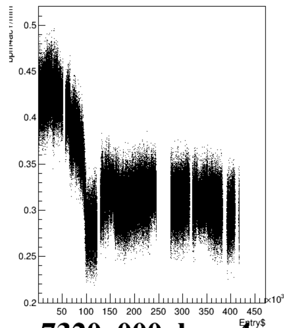
bpm4acY/mm:Entry$ {ErrorFlag==0}
