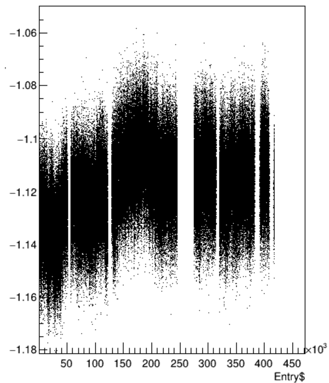
bpm0l01X/mm:Entry$ {ErrorFlag==0}
