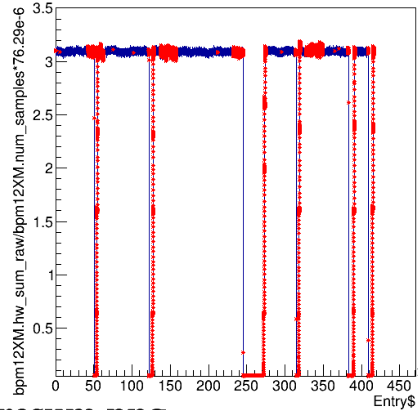
bpm12XM.hw_sum_raw/bpm12XM.num_samples*76.29e-6:Entry$
