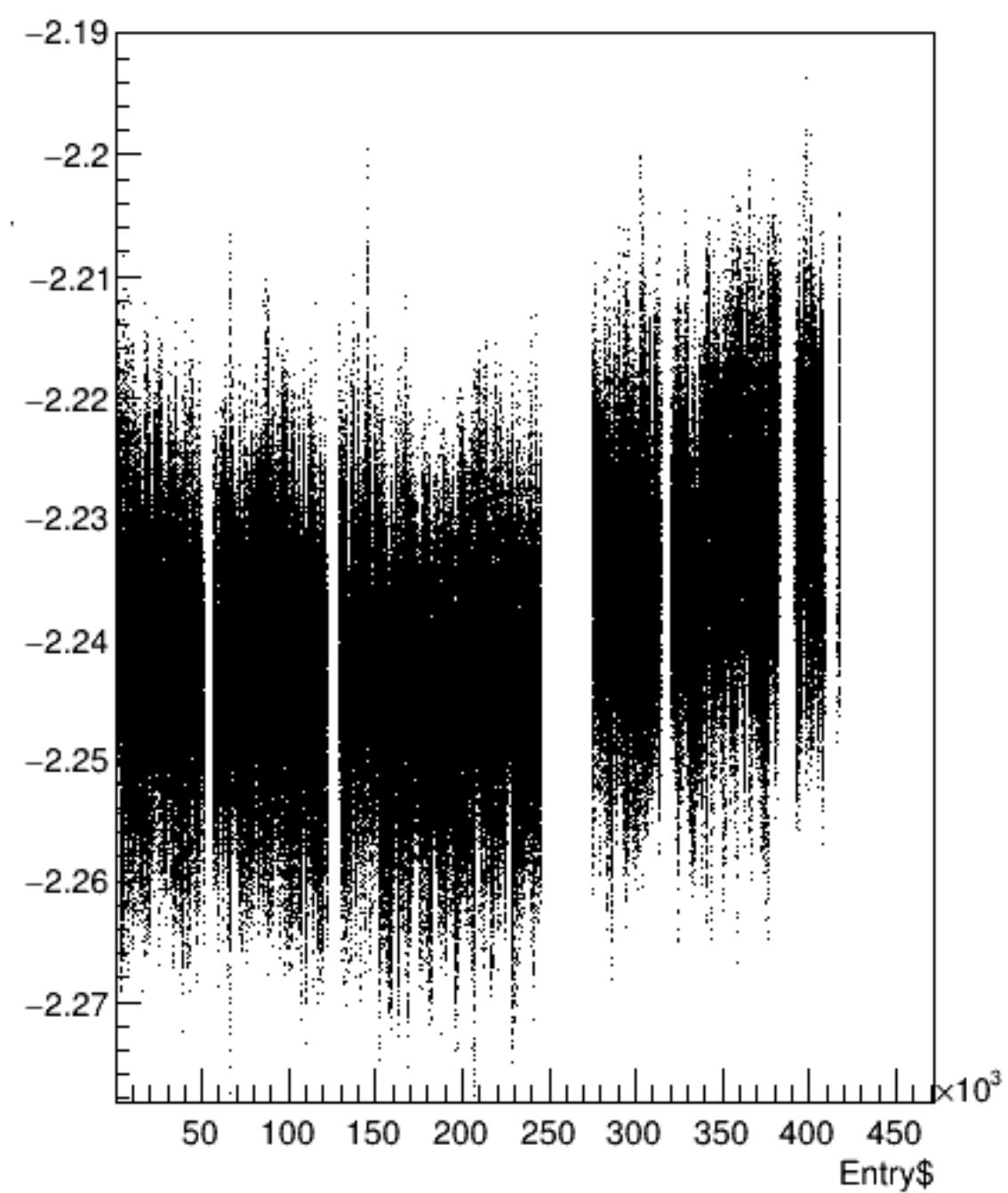
bpm1i02X/mm:Entry$ {ErrorFlag==0}
