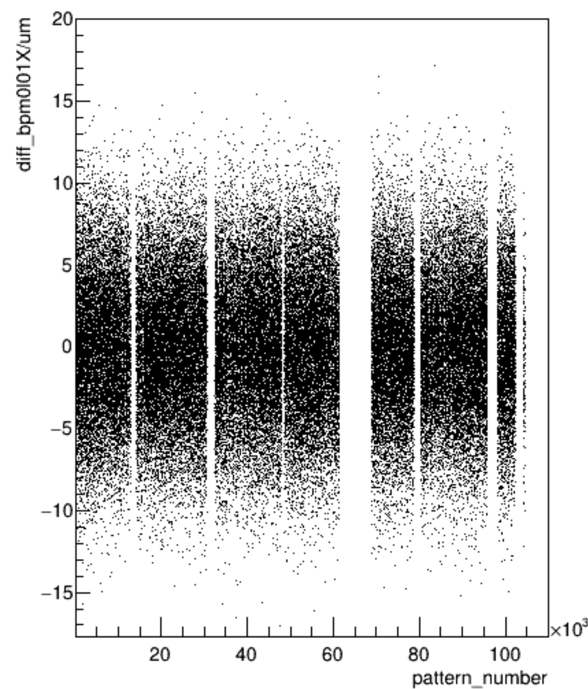
diff_bpm0l01X/um:pattern_number (ErrorFlag==0)
