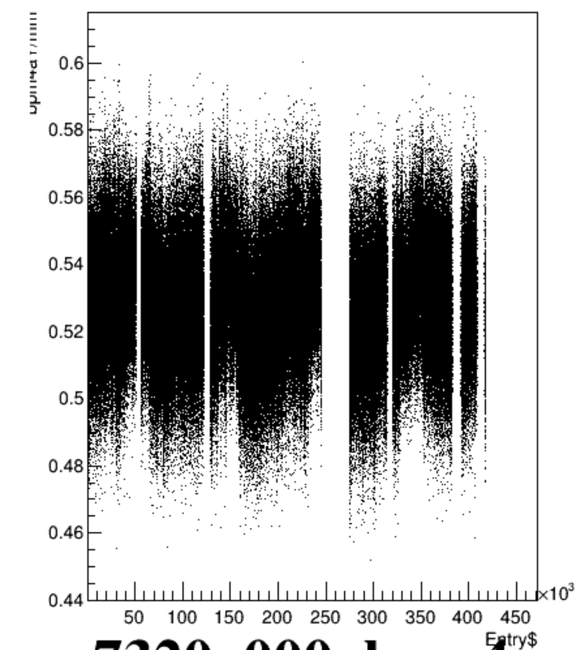
bpm4aY/mm:Entry$ {ErrorFlag==0}
