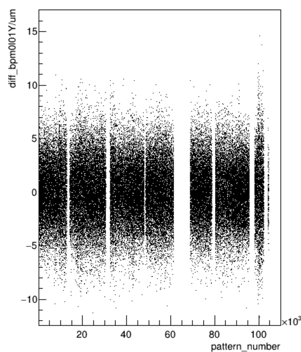
diff_bpm0l01Y/um:pattern_number (ErrorFlag==0)
