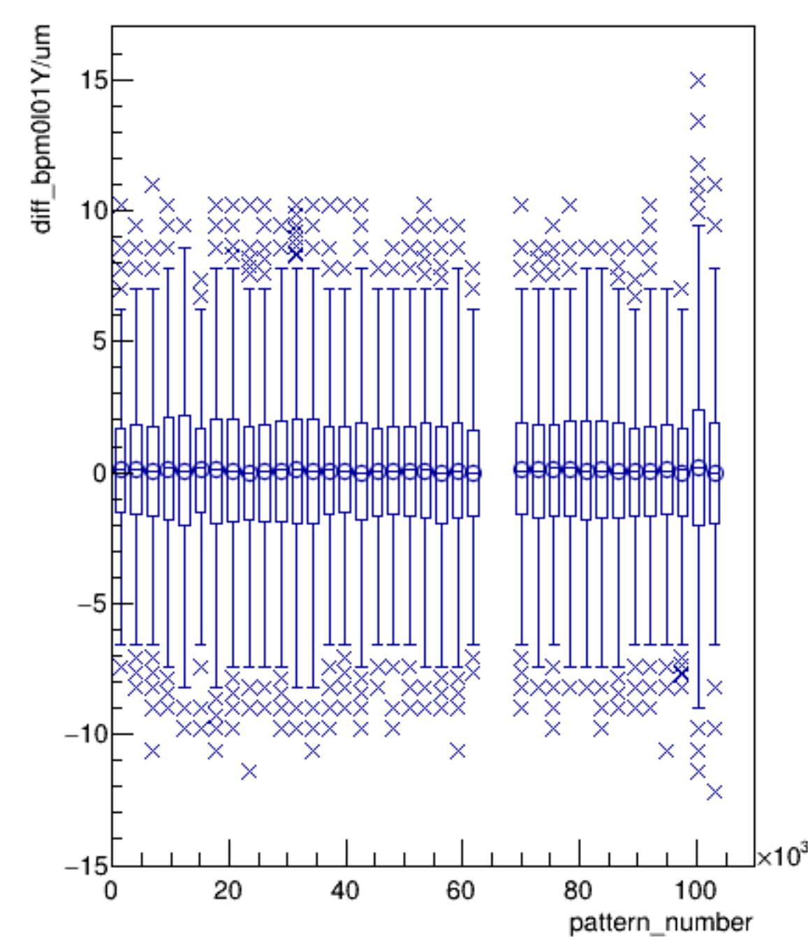
diff_bpm0l01Y/um:pattern_number (ErrorFlag==0)
