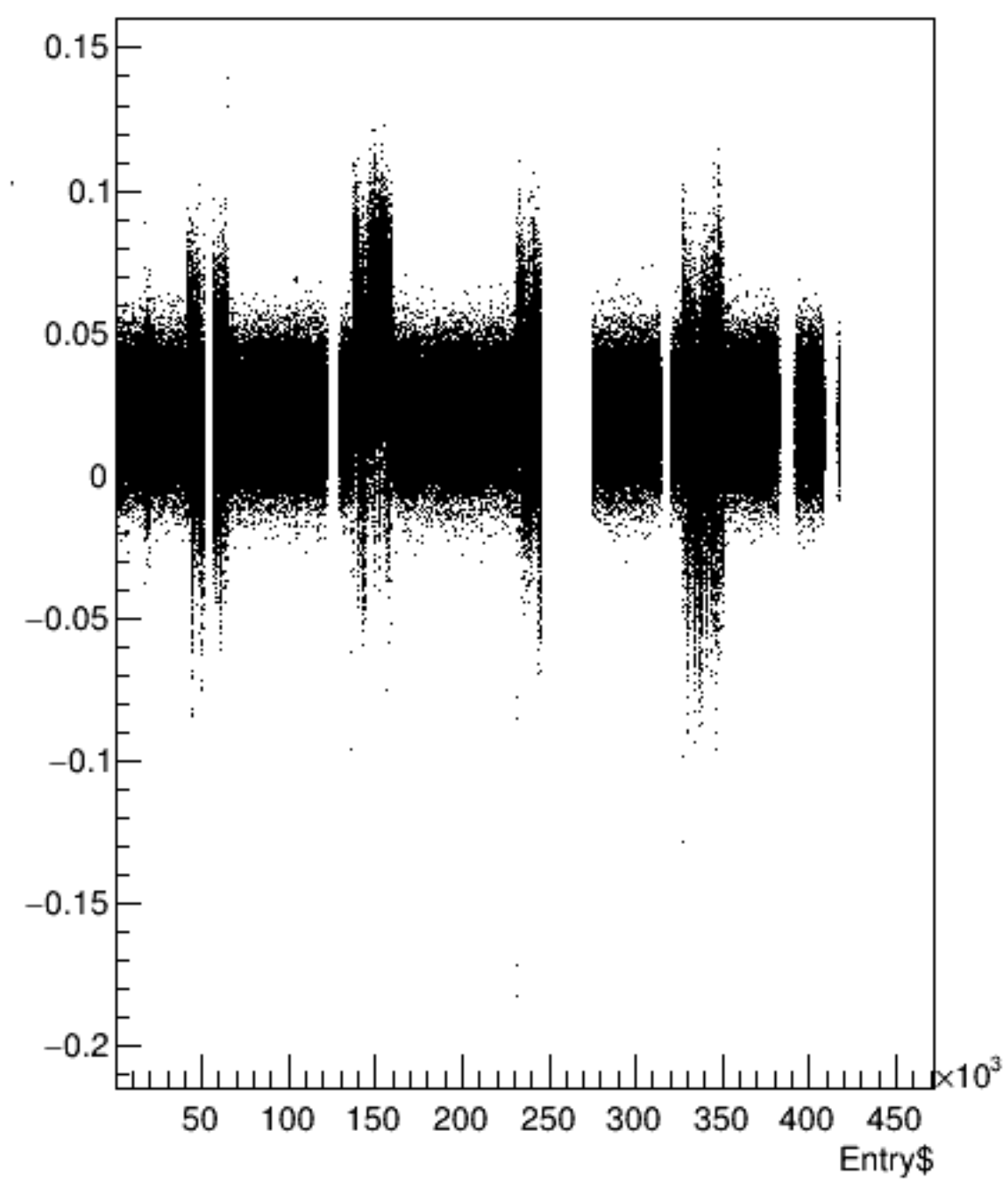
bpm16X/mm:Entry$ {ErrorFlag==0}
