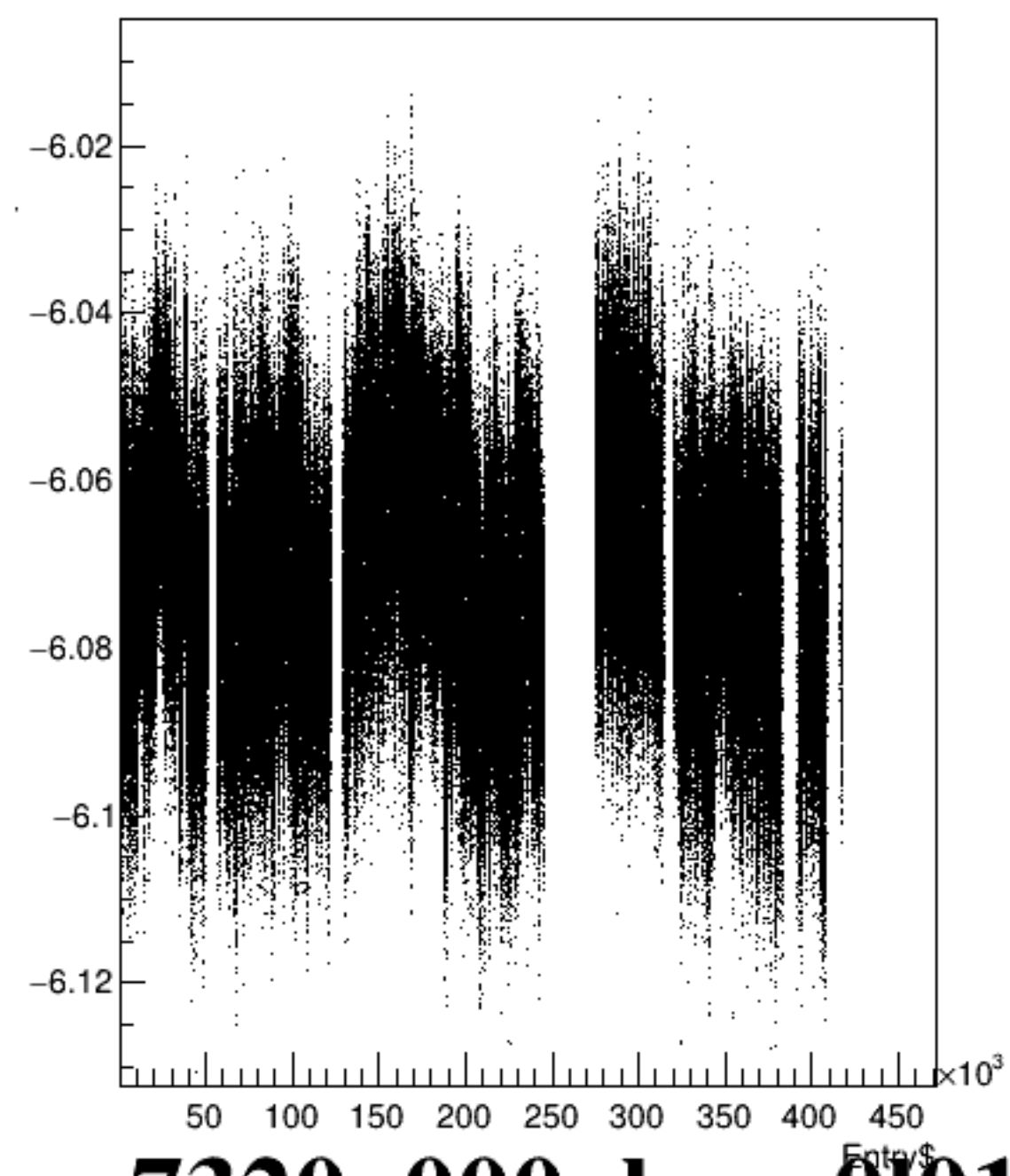
bpm0l01Y/mm:Entry$ {ErrorFlag==0}
