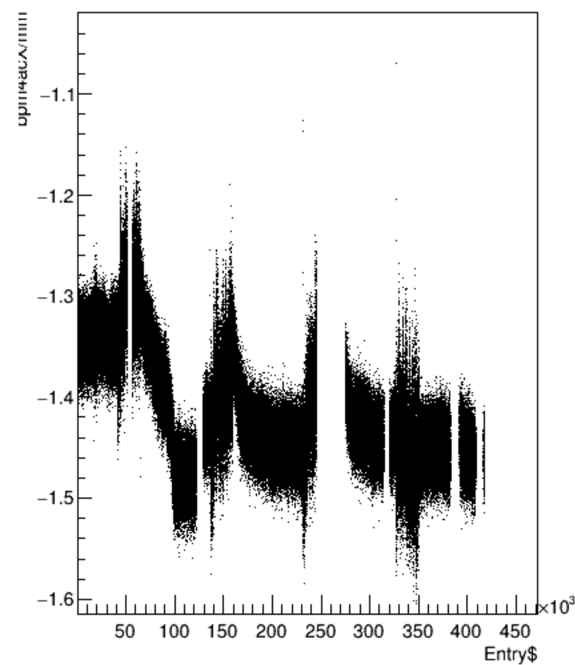
bpm4acX/mm:Entry$ {ErrorFlag==0}
