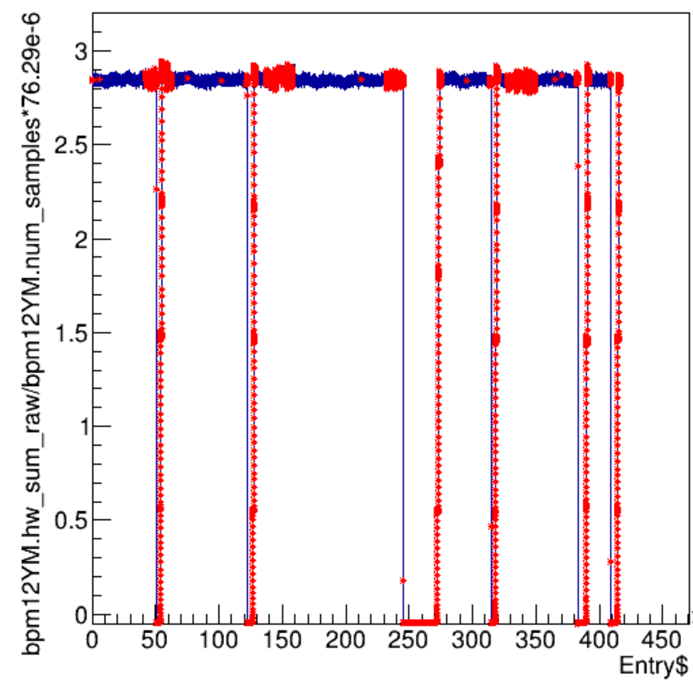
bpm12YM.hw_sum_raw/bpm12YM.num_samples*76.29e-6:Entry$
