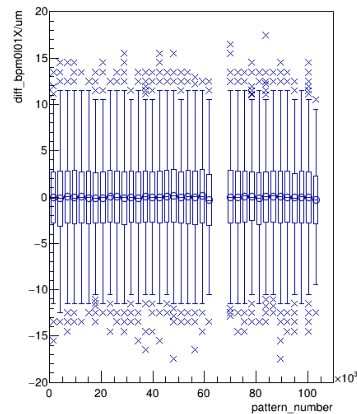
diff_bpm0l01X/um:pattern_number (ErrorFlag==0)
