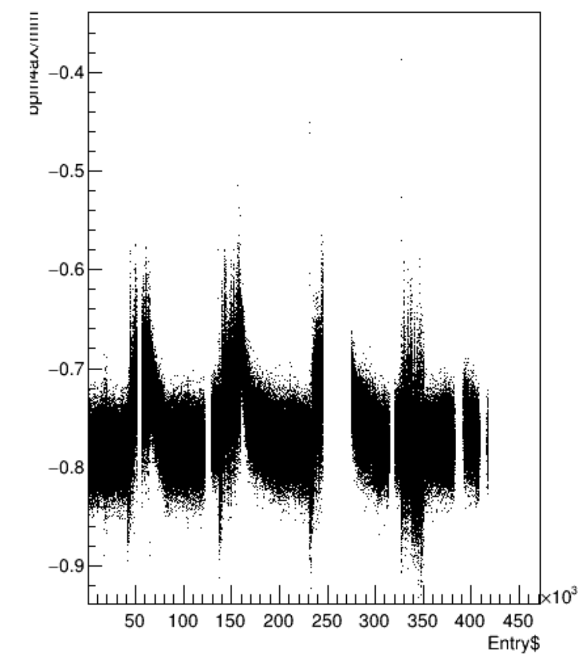
bpm4aX/mm:Entry$ {ErrorFlag==0}
