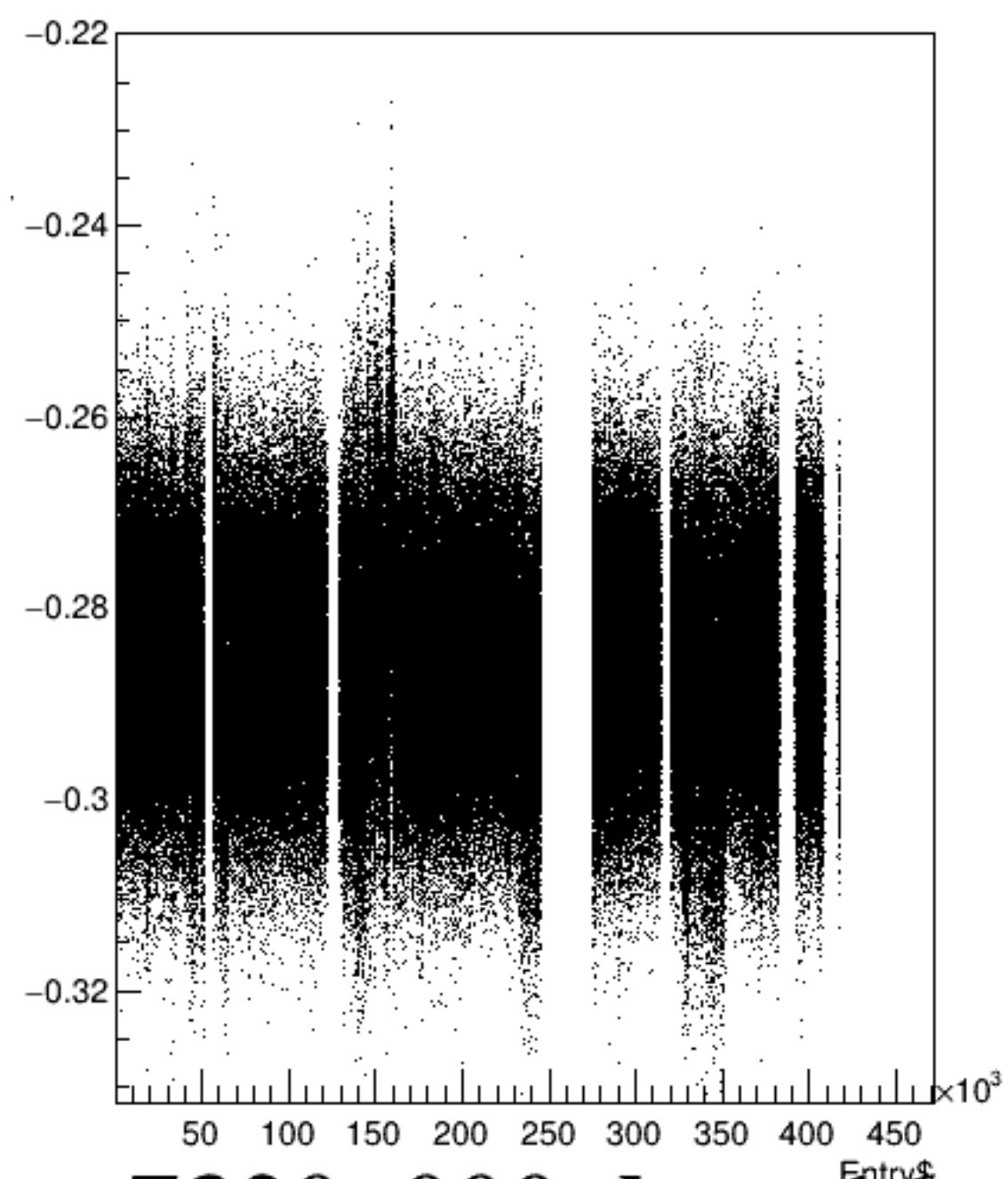
bpm16Y/mm:Entry$ {ErrorFlag==0}
