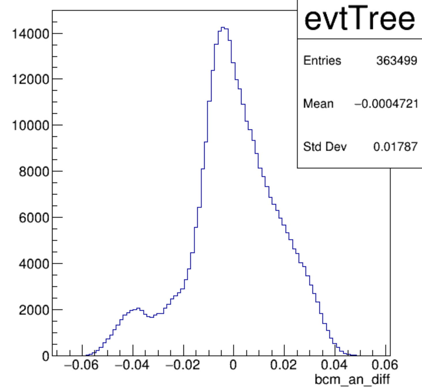
bcm_an_diff {ErrorFlag==0}
