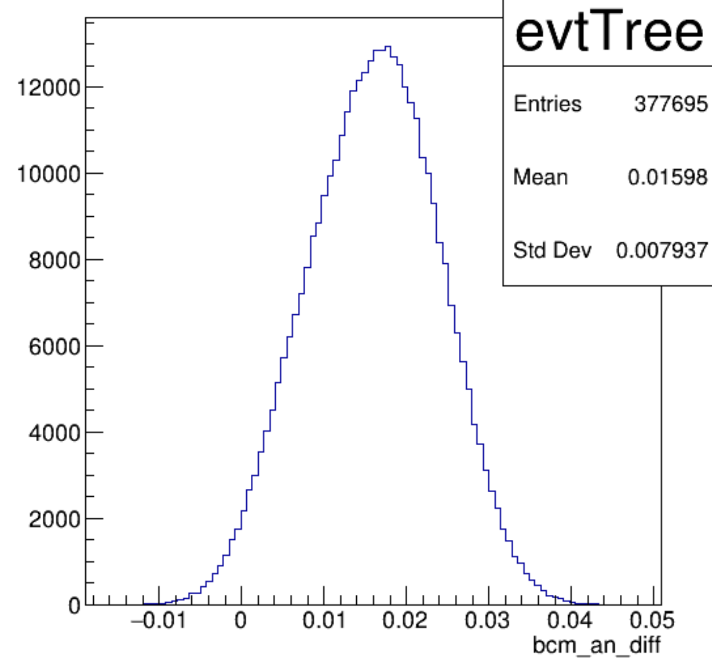
bcm_an_diff {ErrorFlag==0}
