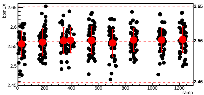
bmod_trim4,cyc=8781
