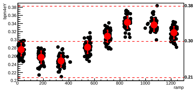
bmod_trim6,cyc=8781
