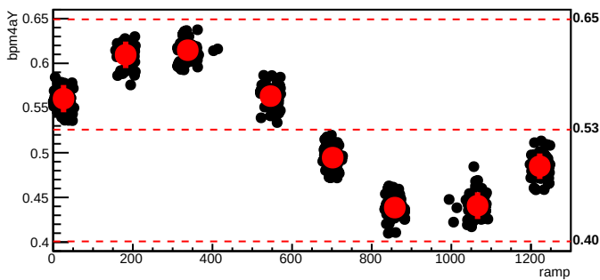
bmod_trim6,cyc=8781
