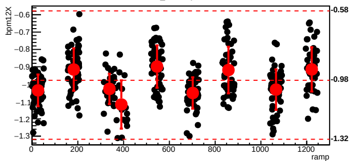
bmod_trim4,cyc=8781
