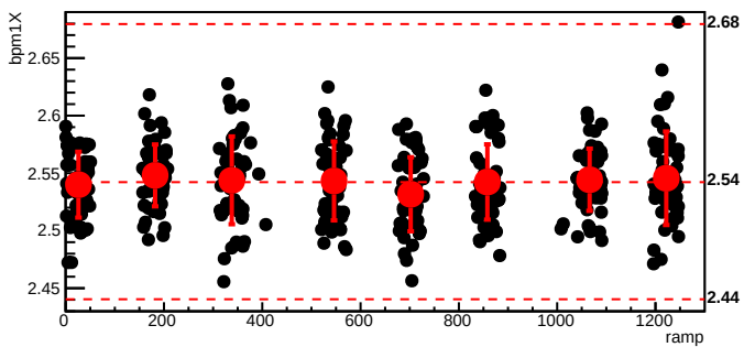
bmod_trim2,cyc=8781
