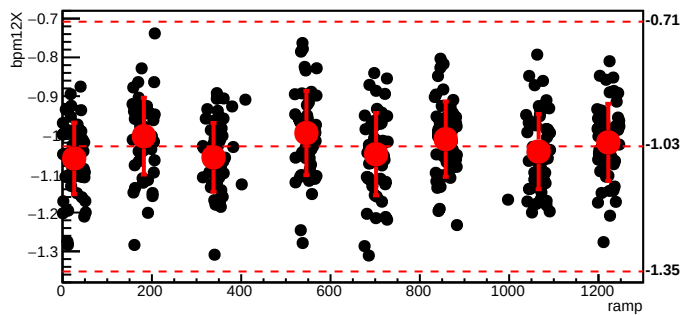
bmod_trim2,cyc=8781
