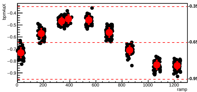
bmod_trim5,cyc=8781
