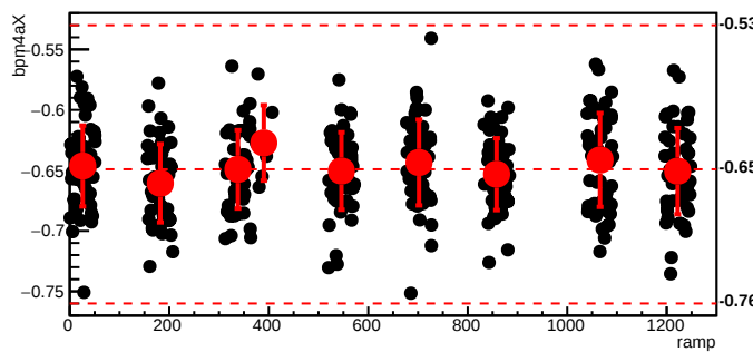
bmod_trim4,cyc=8784
