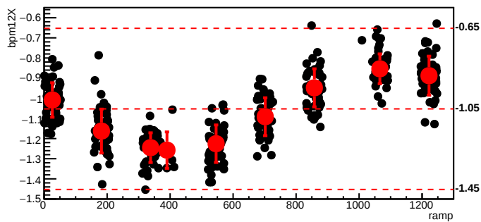
bmod_trim3,cyc=8784
