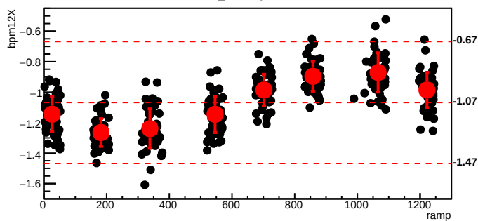
bmod_trim7,cyc=8784
