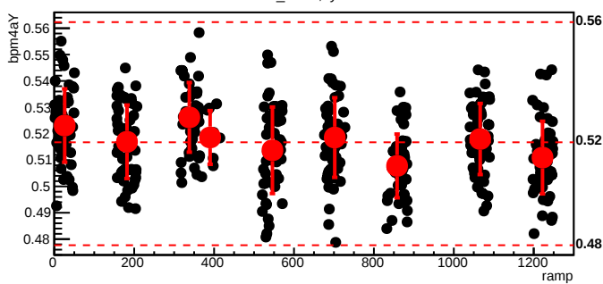
bmod_trim1,cyc=8784
