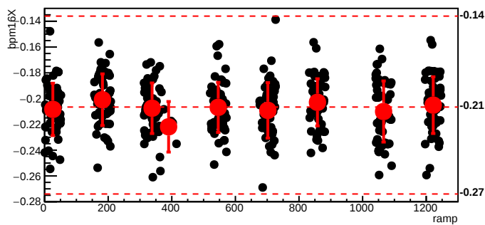
bmod_trim4,cyc=8784
