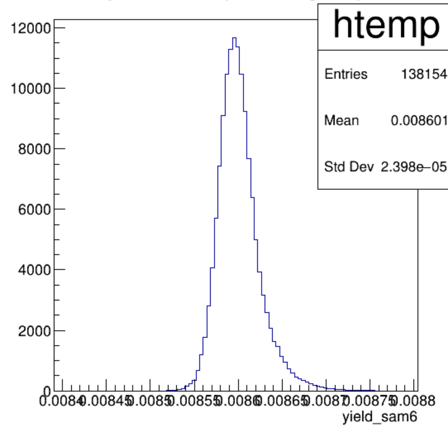
yield_sam6 {ErrorFlag==0}
