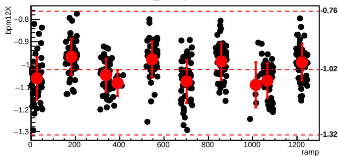
bmod_trim6,cyc=8833
