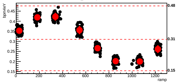
bmod_trim4,cyc=8833
