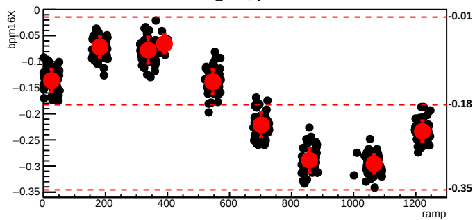
bmod_trim1,cyc=8833
