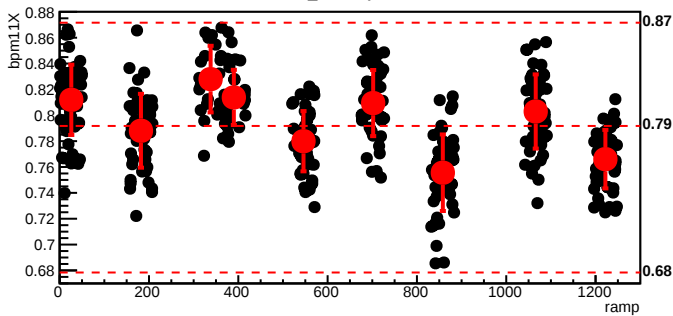
bmod_trim6,cyc=8867
