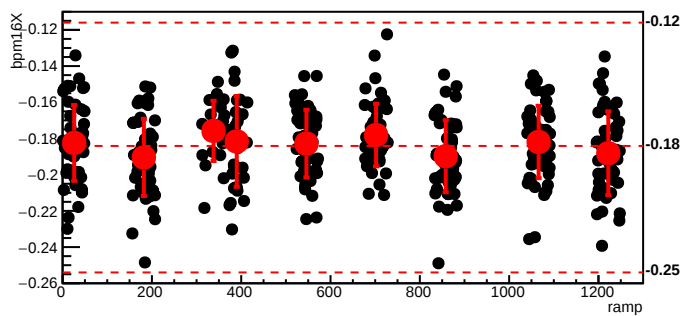
bmod_trim4,cyc=8867
