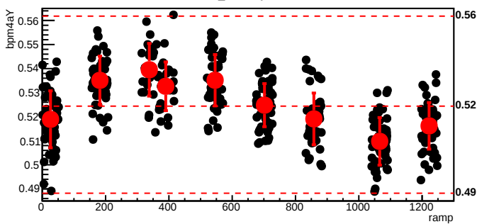
bmod_trim3,cyc=8867
