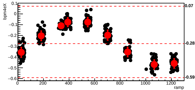
bmod_trim5,cyc=8867
