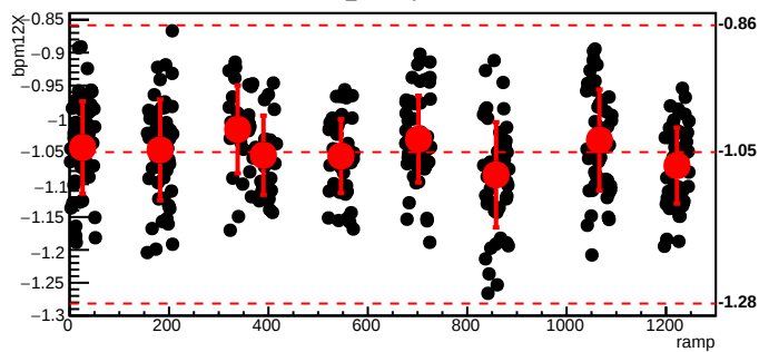
bmod_trim6,cyc=8867
