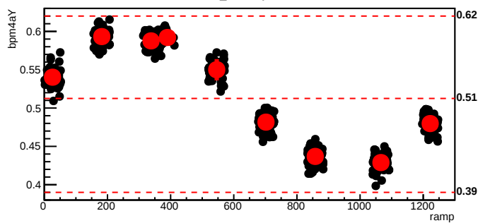
bmod_trim2,cyc=8867
