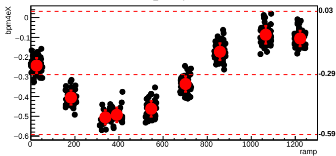
bmod_trim3,cyc=8867
