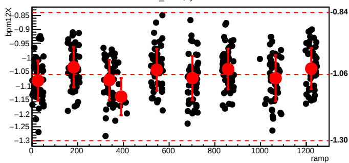
bmod_trim4,cyc=8943
