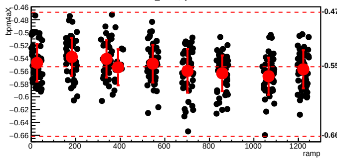
bmod_trim7,cyc=8943
