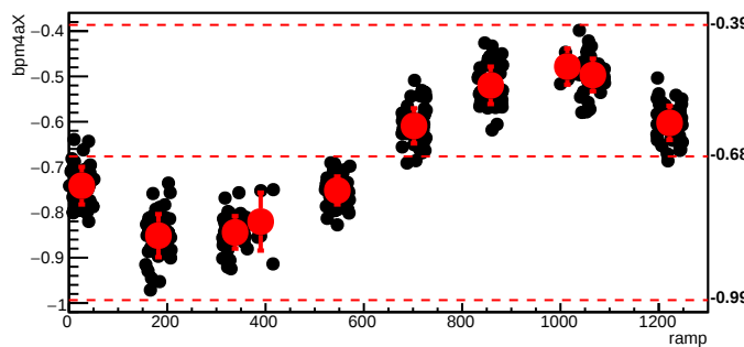
bmod_trim1,cyc=8943
