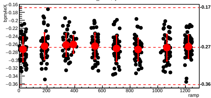
bmod_trim2,cyc=8943
