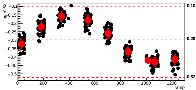
bmod_trim3,cyc=8943
