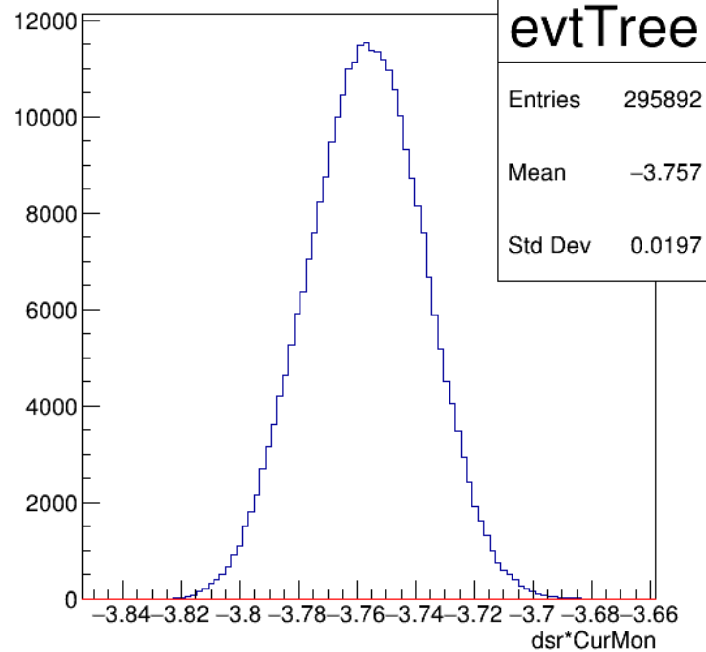
dsr*CurMon {ErrorFlag==0}
