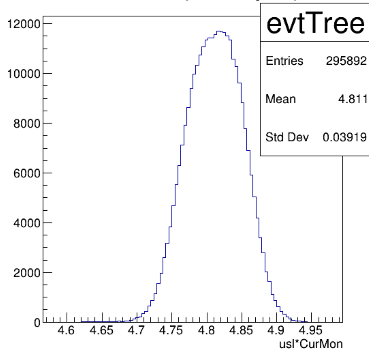
usl*CurMon {ErrorFlag==0}
